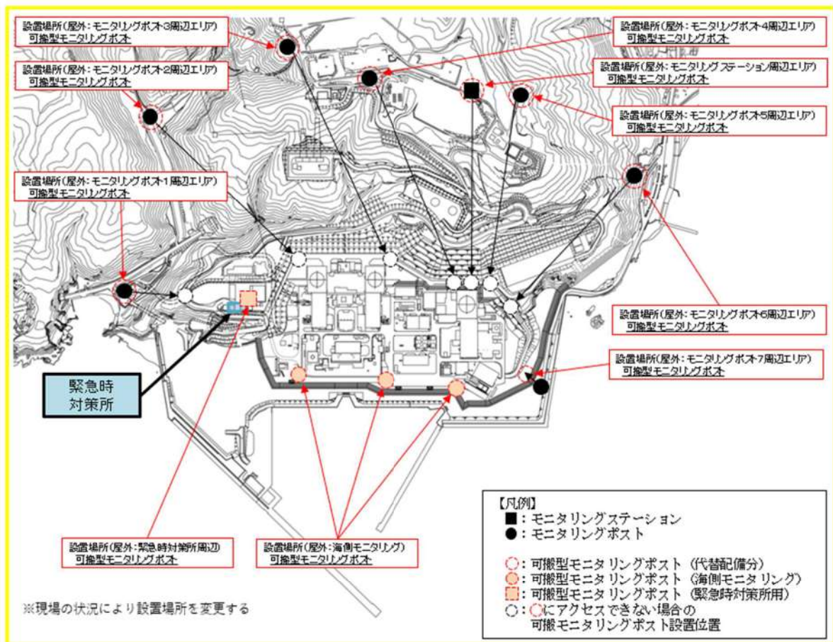
図添 14-2 プルूमの状況を検知する手段
