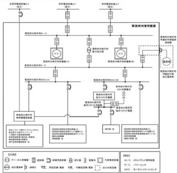
第2.2-1図 緊急時対策所 単線結線図
