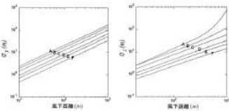
(a) y 方向の拡がりのパラメータ \sigma_y (b) z 方向の拡がりのパラメータ \sigma_z
