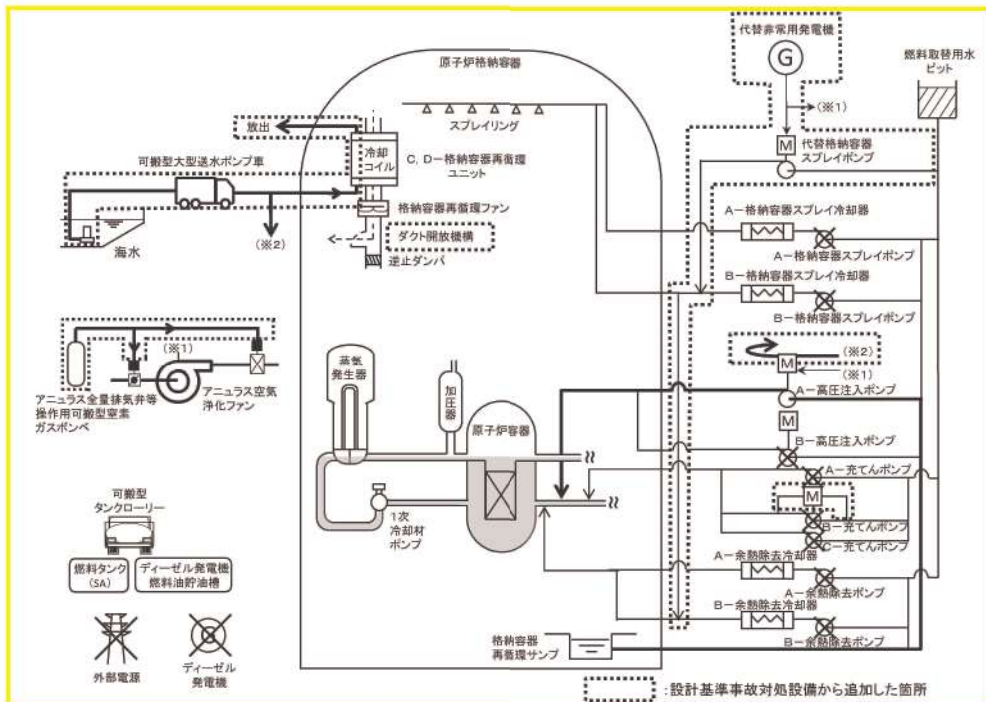
図2 「燃料取出前のミッドループ運転中に外部電源が喪失するとともに非常用所内交流電源が喪失し、原子炉補機冷却機能が喪失する事故」の重大事故等対策の概略系統図（高压代替再循環及び格納容器内自然対流冷却）
