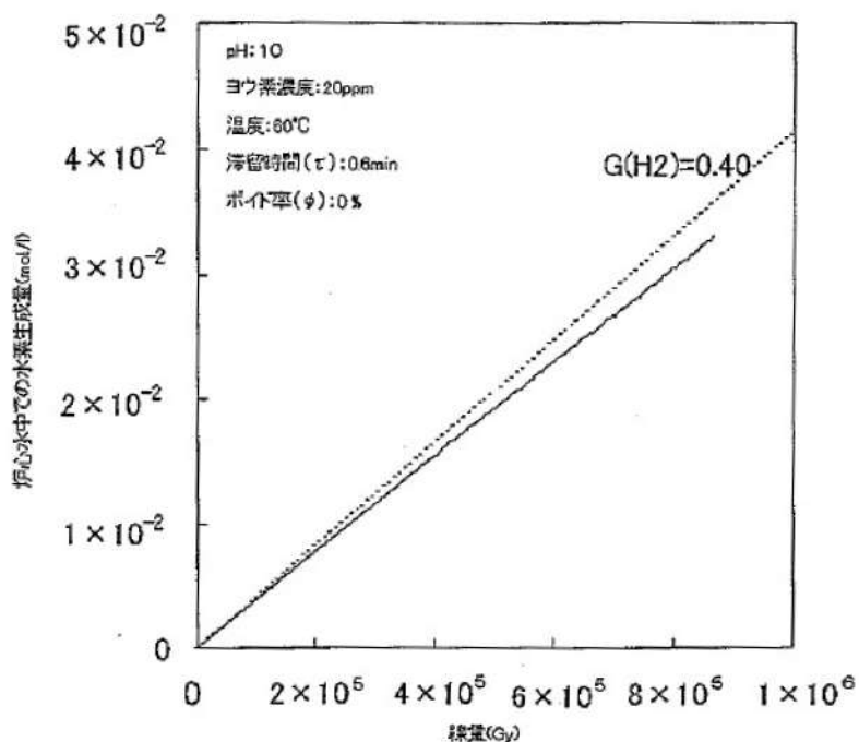
図3.2-9 実効G値への吸収線量の影響(非流動)
