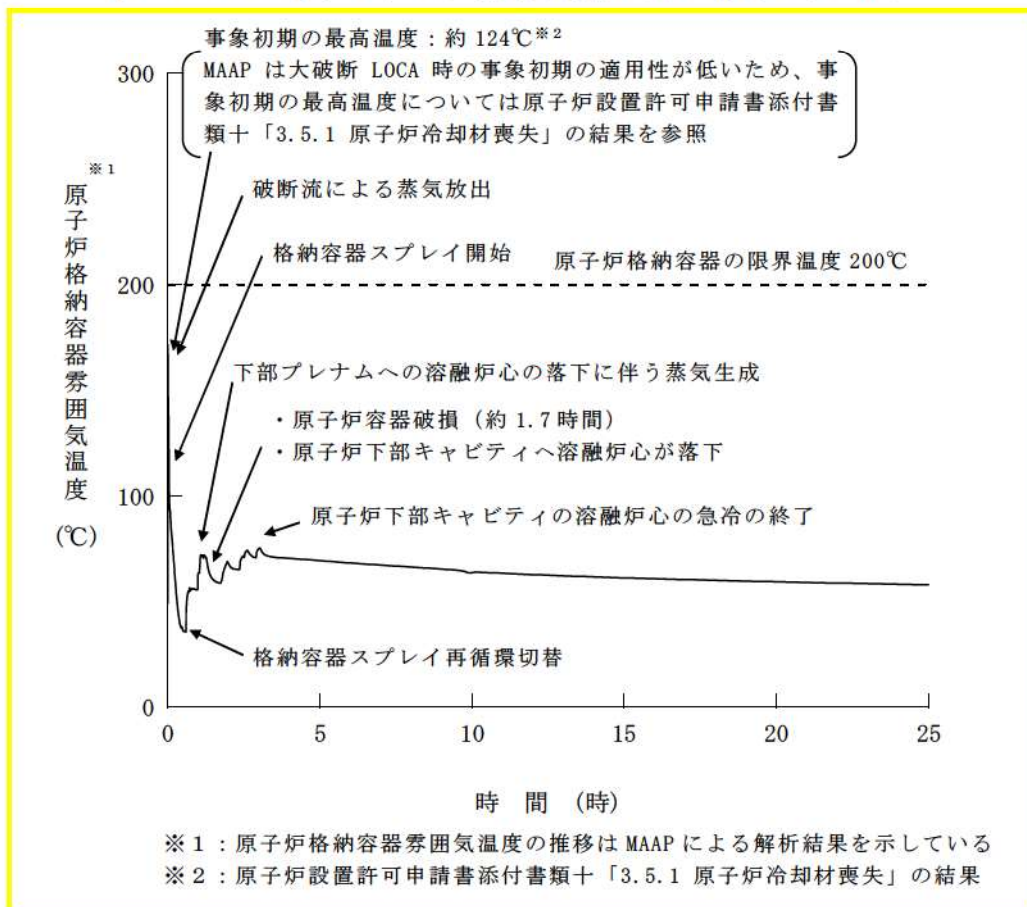
第 7.2.4.14 図 原子炉格納容器雰囲気温度の推移 (MAAP)
