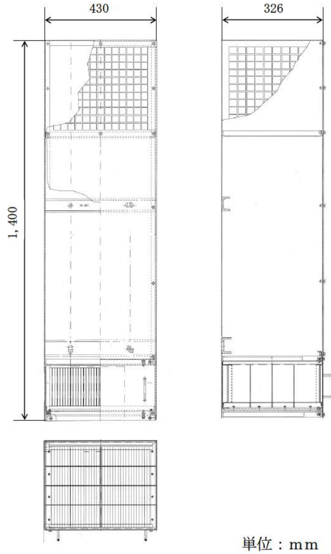
図 40 PARの構造
