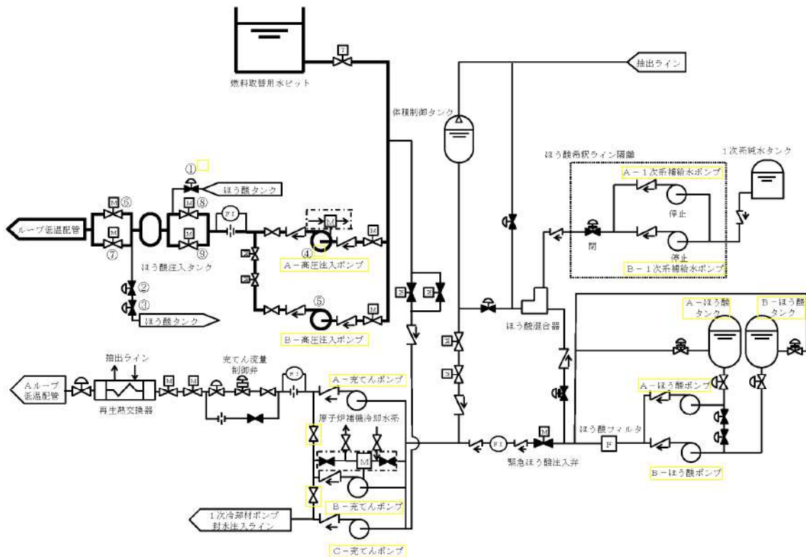
図 44-9-3 高圧注入ポンプ、燃料取替用水ピット及びほう酸注入タンクを用いたほう酸水注入の概要図
