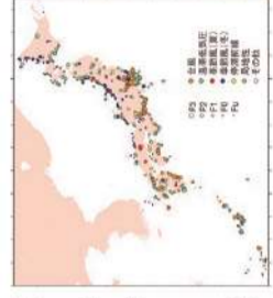
図3 総観場分布
