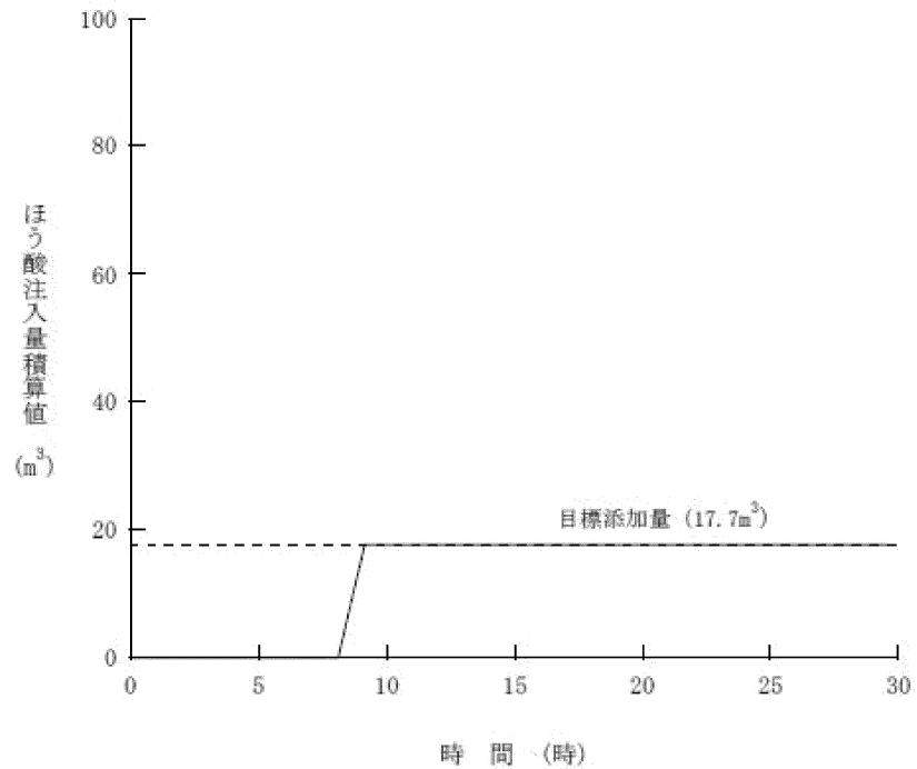
ほう酸注入量積算値の推移 (SBO+LUHS+蓄圧注入失敗+RCP-SDS正常作動)
