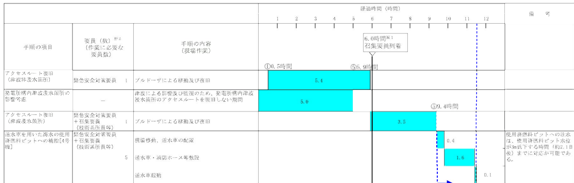
第 3.1.4.3.1.6 図 使用済燃料ピットへの送水車による海水注水の対応手順と所要時間
