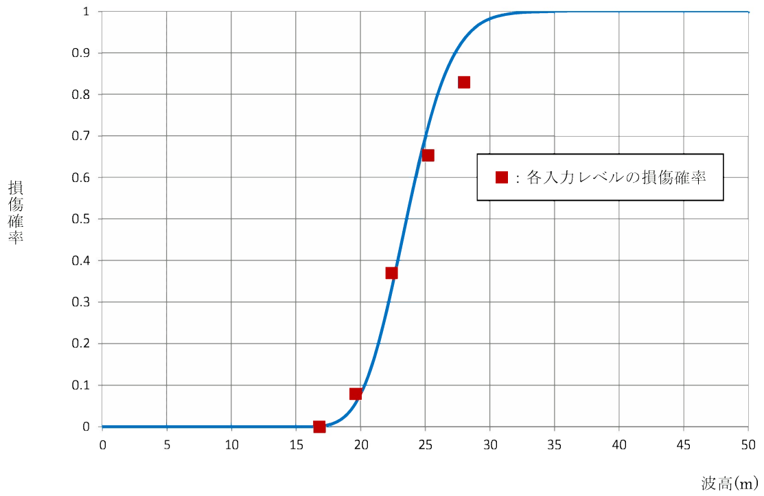
第 3.1.3.2.2.3.8 図 詳細法による fragility 曲線（復水タンク：漂流物）
