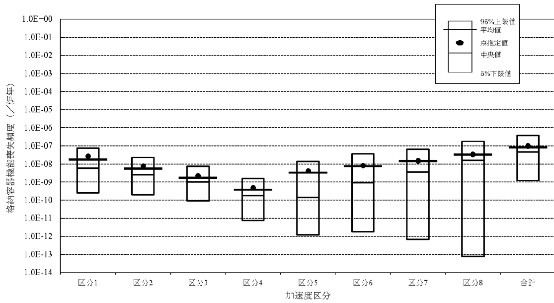
第 3.1.3.2.1.5.3 図 格納容器機能喪失頻度の不確かさ解析結果 (加速度区分別)
