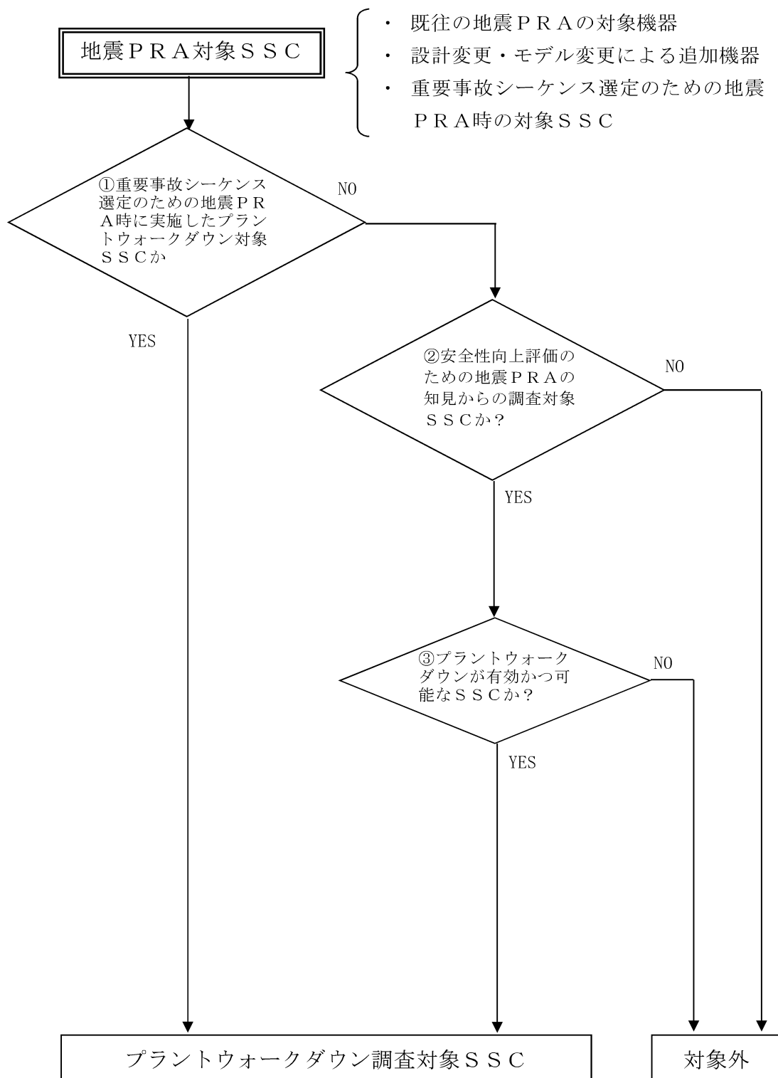
第 3.1.3.2.1.1.1 図 プラント・ワークダウン調査SSCの選定フロー
