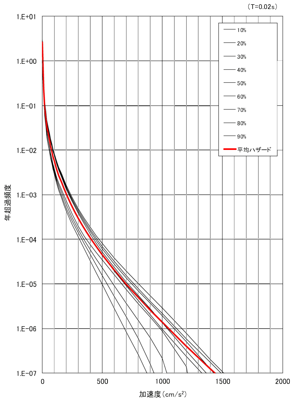
第 3.1.3.2.1.2.8 図 フラクタル地震ハザード曲線 (周期 0.02 秒)
