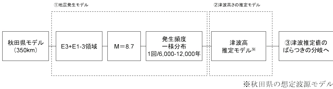
第 3.1.3.2.2.9 図 日本海東縁部（秋田県）の地震発生・津波高推定モデル
