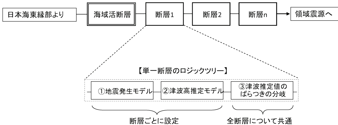
第 3.1.3.2.2.10 図 海域活断層のロジックツリー
