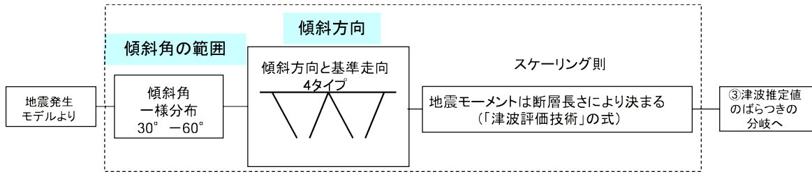
第 3.1.3.2.2.8 図 日本海東縁部（土木学会）の津波高推定モデル
