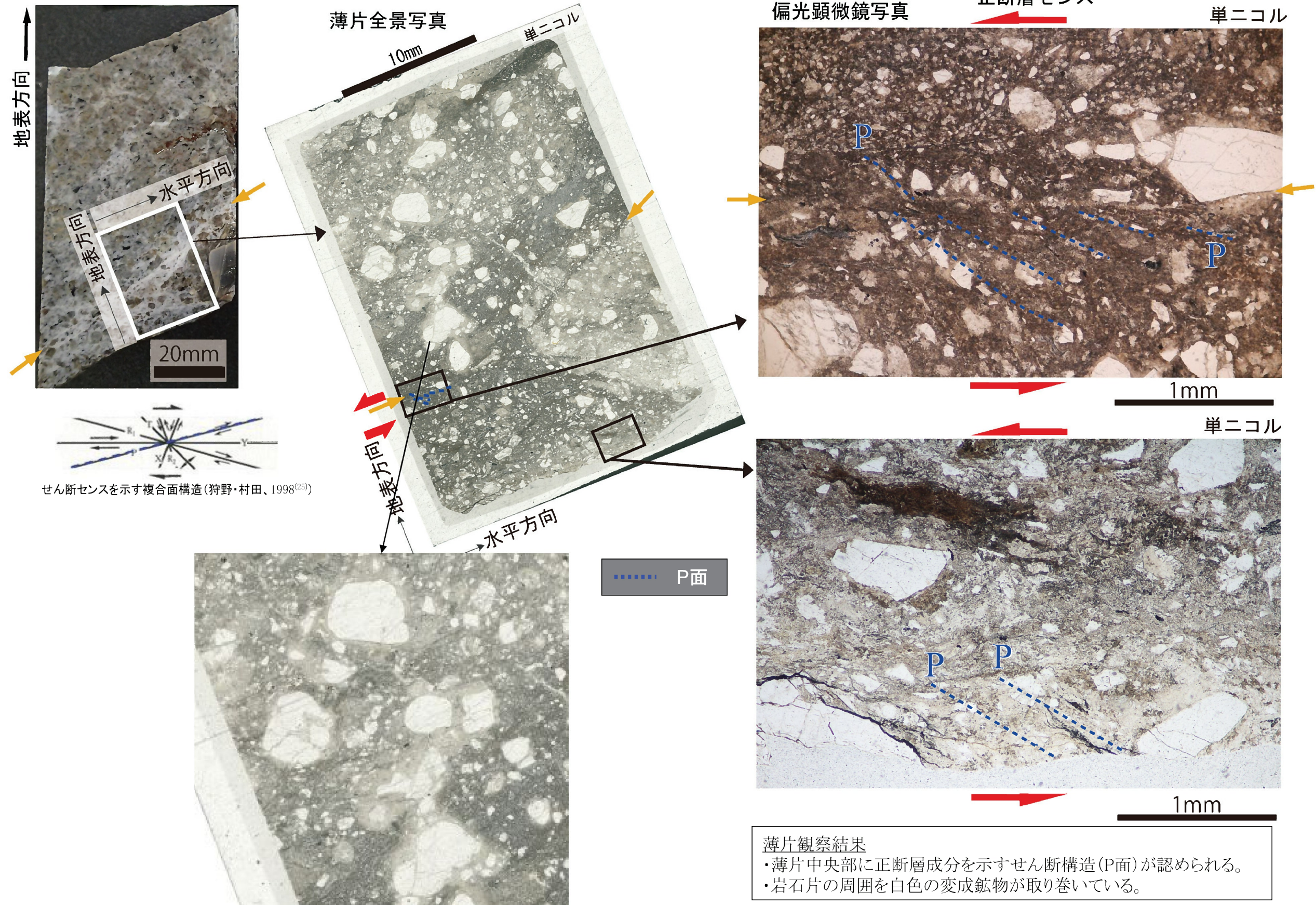
第1.2.3.4.17図 F-C (T3-6孔) 薄片観察結果
