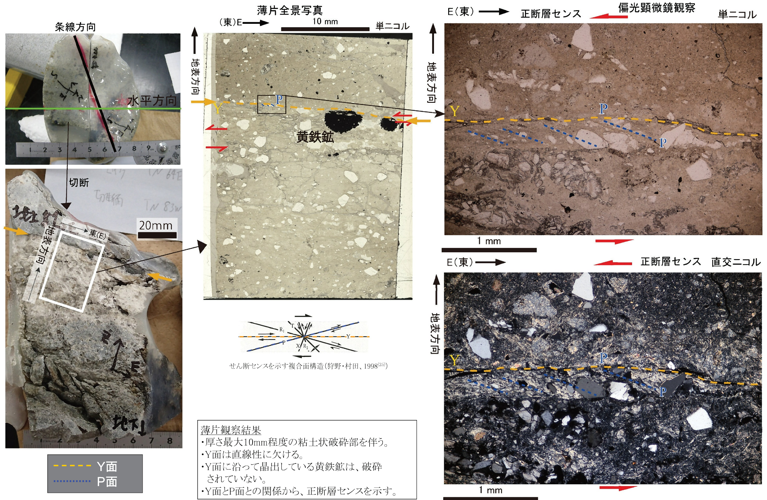
第1.2.3.4.15図 F-C (H25-9孔破碎部2) 薄片観察結果
