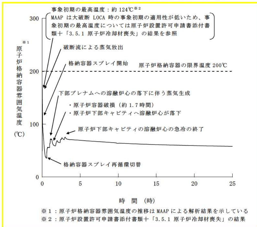
第 7.2.4.14 図 原子炉格納容器雰囲気温度の推移 (MAAP)
