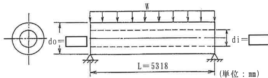
(口)-第 A. 30 図 両端単純支持された容器の解析モデル図
