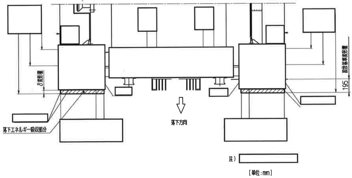
(口)-第 A. 16 図 水平落下解析モデル
