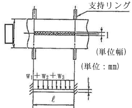
(口)-第 A. 49 図 チャンネル板 水平落下時の解析モデル
