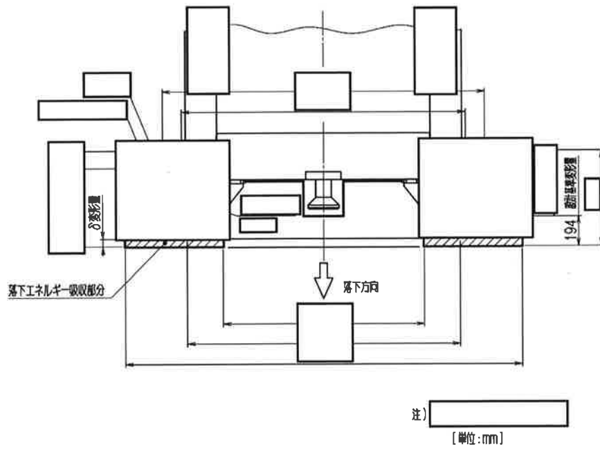
(口)-第 A. 12 図 頭部垂直落下解析モデル
