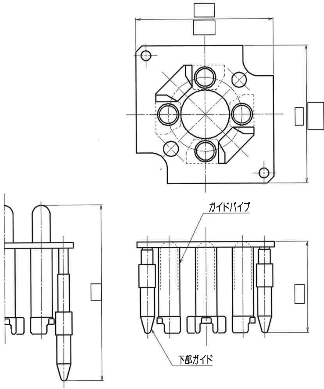
ばね収縮時
