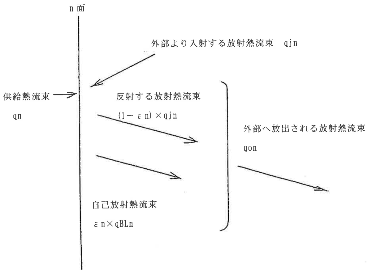
(口)-第 B. 付 4 図 n 面での放射
