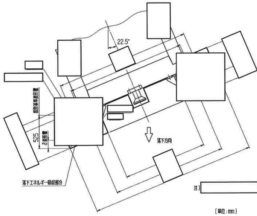
(口)-第 A. 18 図 頭部コーナー落下解析モデル
