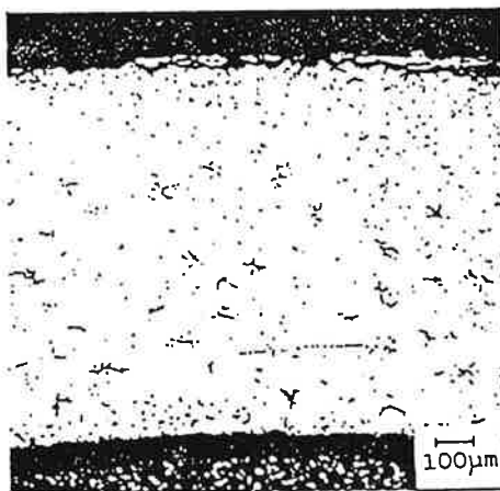
写真4 被覆管横断面水素化物の金相写真
