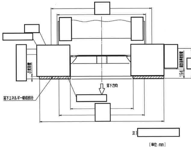
(口)-第 A. 14 図 底部垂直落下解析モデル
