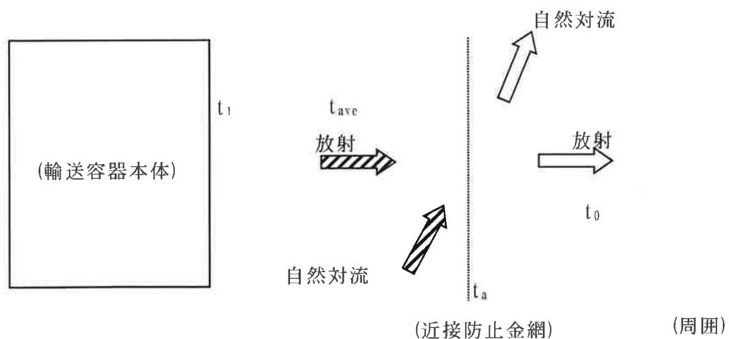
(□)-第 B. 付 8 図 近接防止金網周りの伝熱モデル
