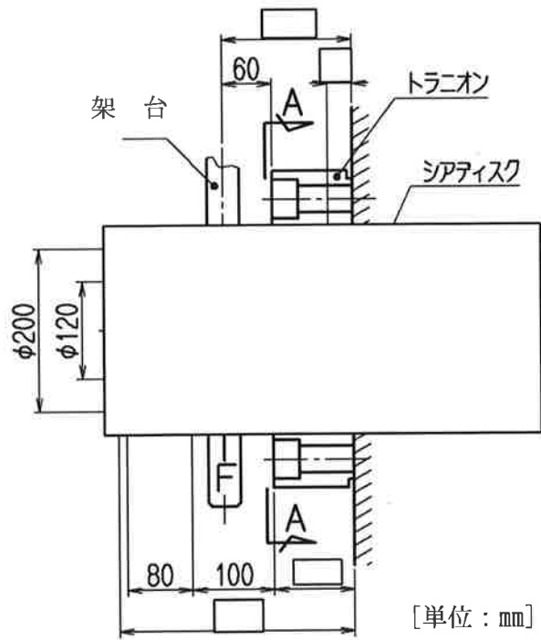
(口)-第 A. 5 図 輸送架台固縛状態解析モデル図
