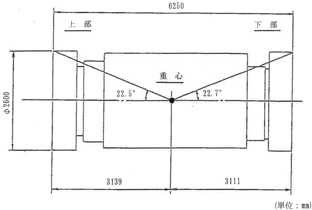
(口)-第A.1図 重心の位置
