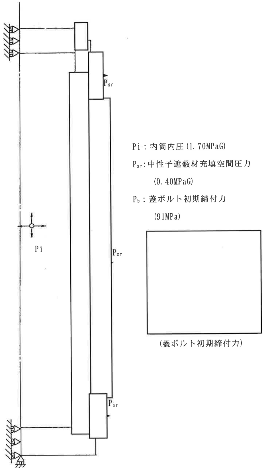
(口)-第 A. 8 図 一般の試験条件の熱的試験における荷重条件及び境界条件
