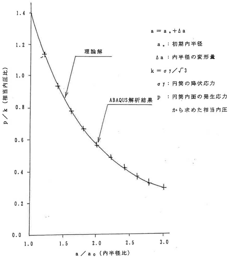
(口)-第A.参2図 ABAQUS コードの検証例
