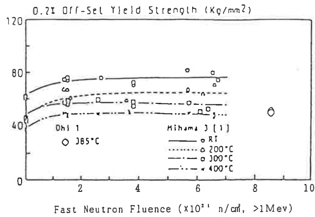
(口)-第A. 参 12 図 ジルカロイの耐力の中性子照射量に対する変化 (PWR) 3)
