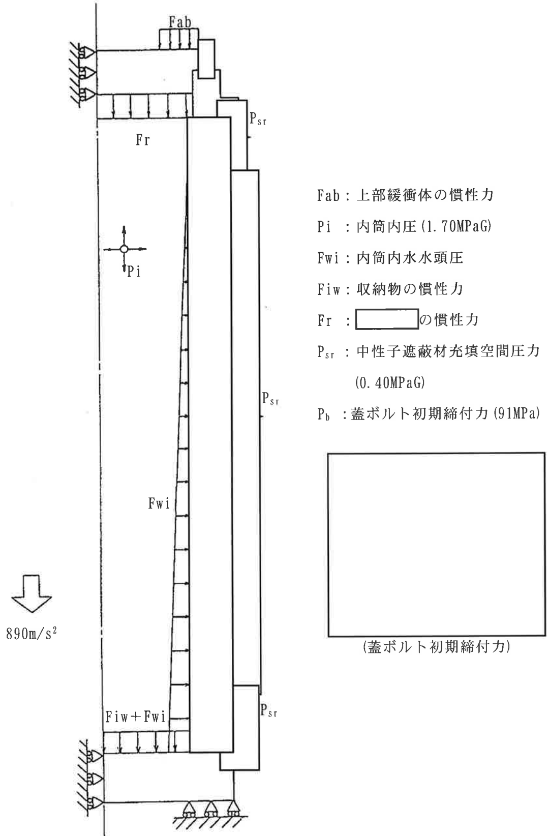
(口)-第 A. 44 図 底部 9m 垂直落下時の荷重条件及び境界条件
