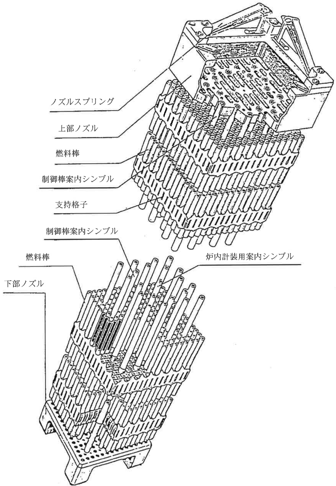
(イ)-第D.1図 PWR 燃料集合体全体図
