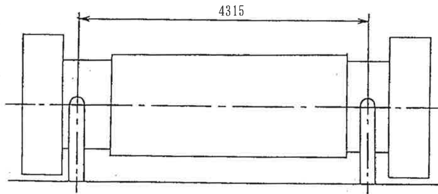
(口) - 第 A. 6 図 輸送架台モデル図
