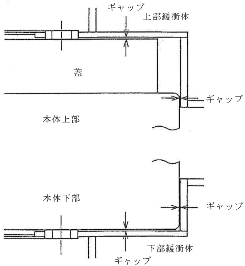
(口)-第 B. 付 7 図 緩衝体と容器本体のギャップ
