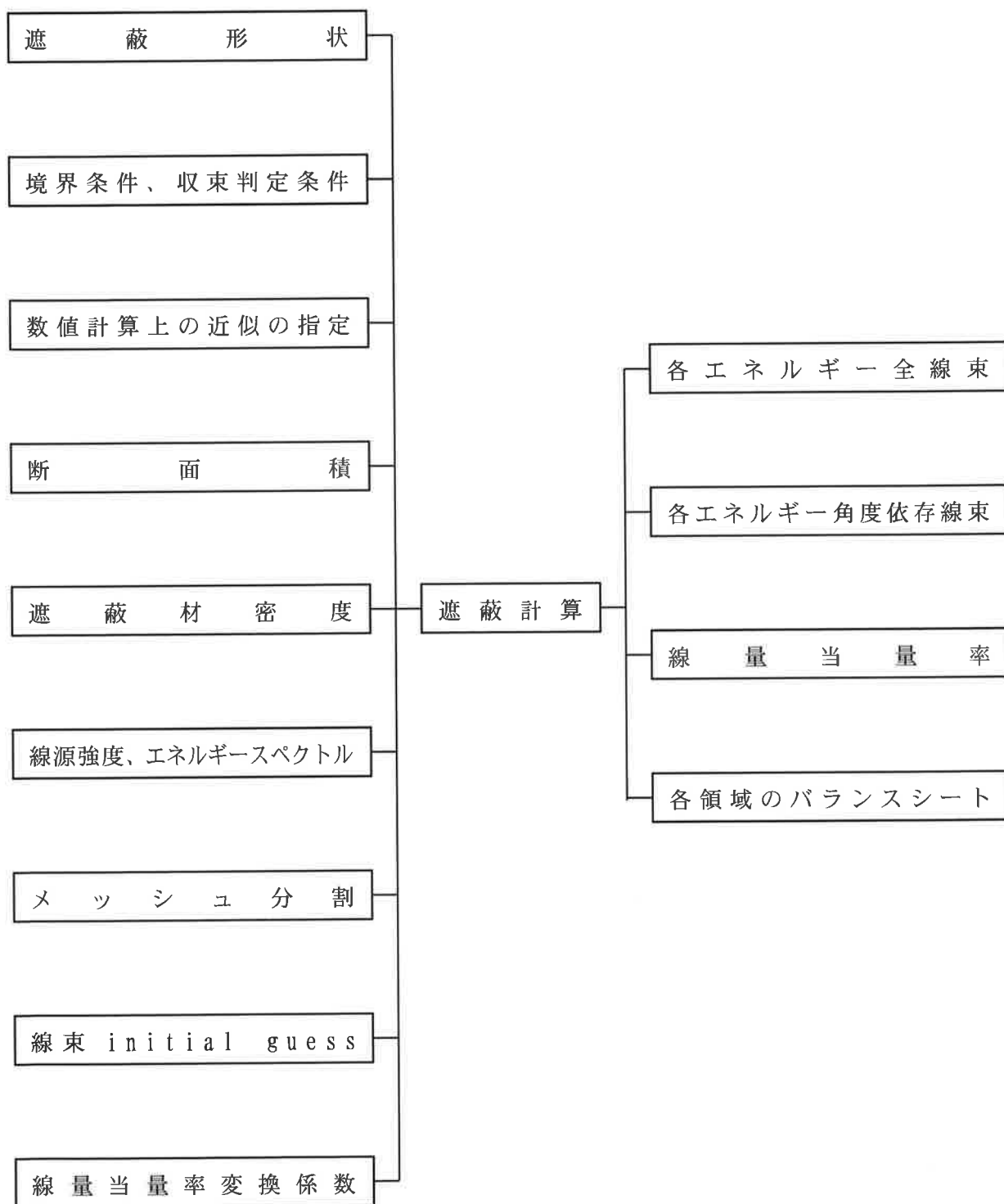
(口)-第D. 参3図 DOT3.5 コード インプット/アウトプット
