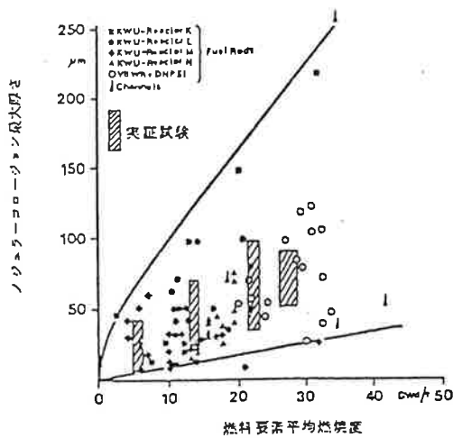
第10図 ノジュラーコロージョン最大厚さの燃焼度変化
