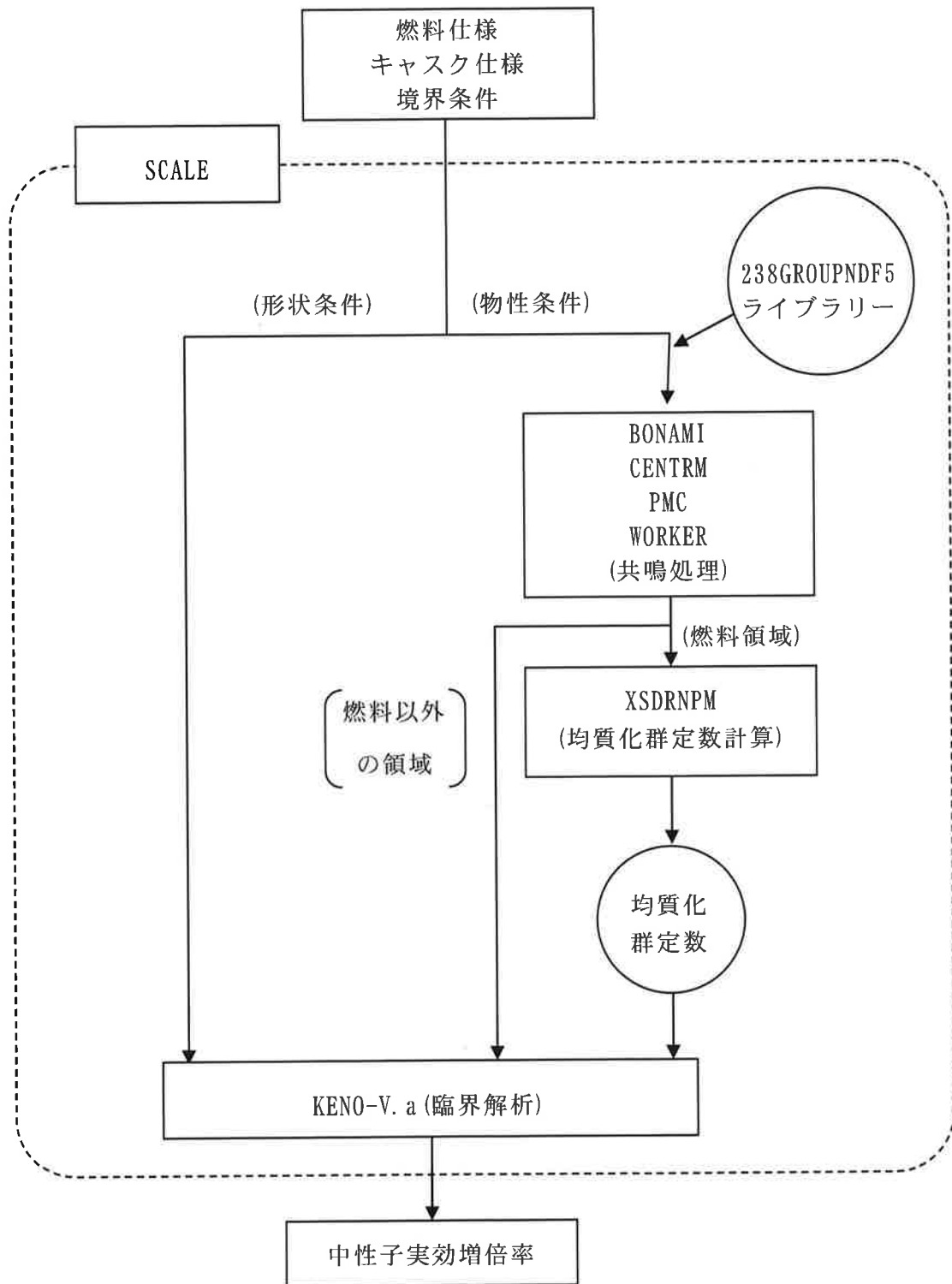
(口)-第 E. 3 図 臨界計算の流れ
