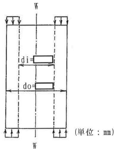
(口)-第 A. 31 図 両端より圧縮される容器の解析モデル
