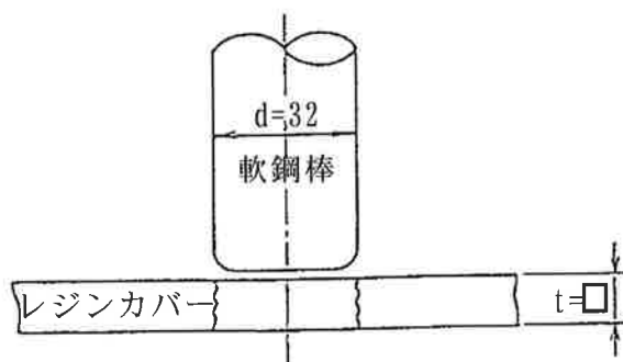
(口)-第 A. 32 図 せん断による貫通モデル図
