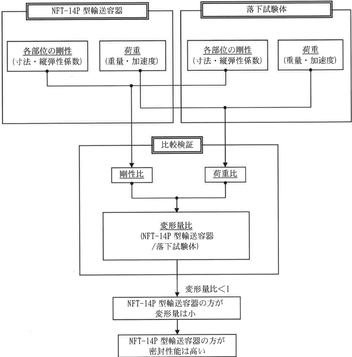
(□)-第 A. 付 19 図 密封性能評価手順
