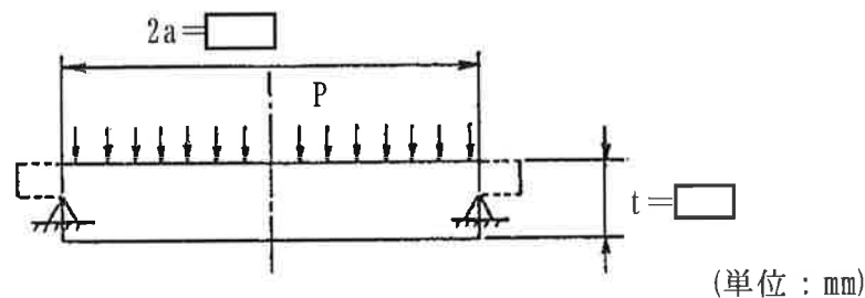
(口)-第 A. 55 図 外圧に対する蓋の強度解析モデル
