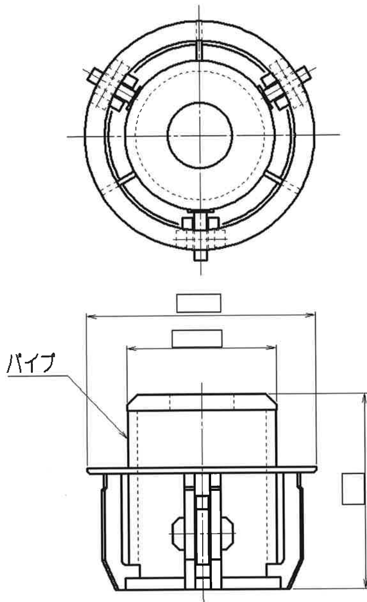
(イ)-第D.15図 下部スツール
