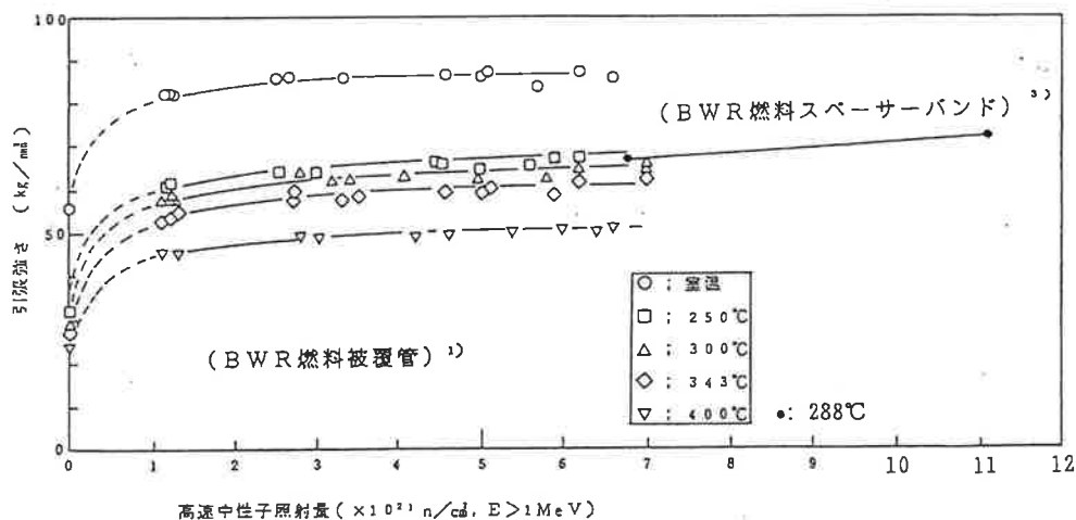
(ロ)-第A. 参10 図 ジルカロイの引張強さの中性子照射量に対する変化 (BWR)
