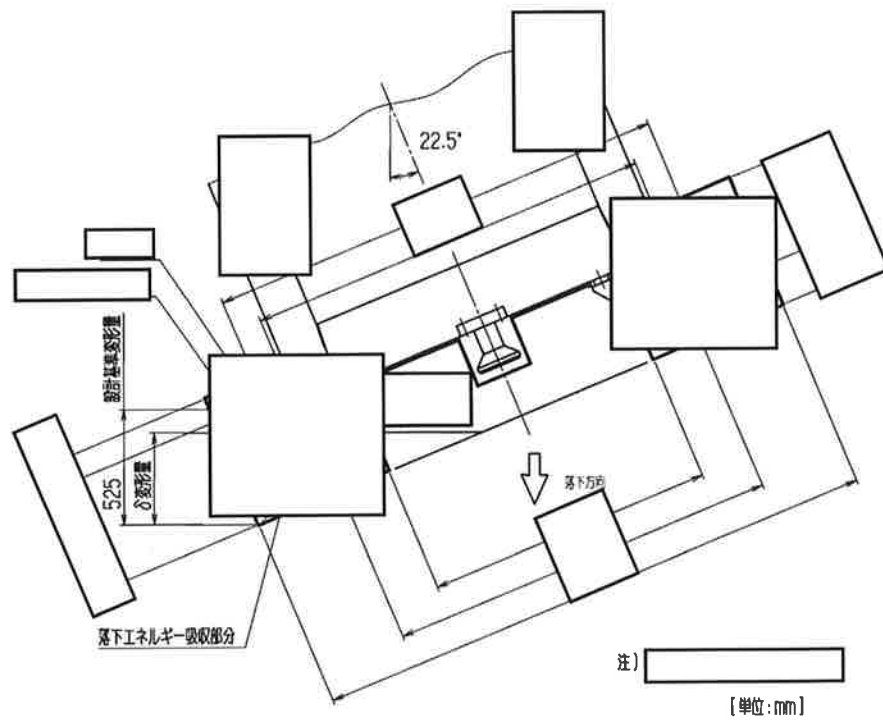
(口)-第 A. 39 図 頭部コーナー落下解析モデル
