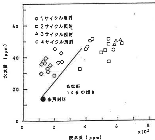
第12図 被覆管中の水素量：酸素量
