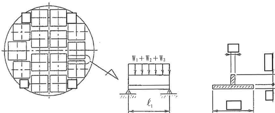
(□)-第 A. 50 図 チャンネル支持部解析モデル
