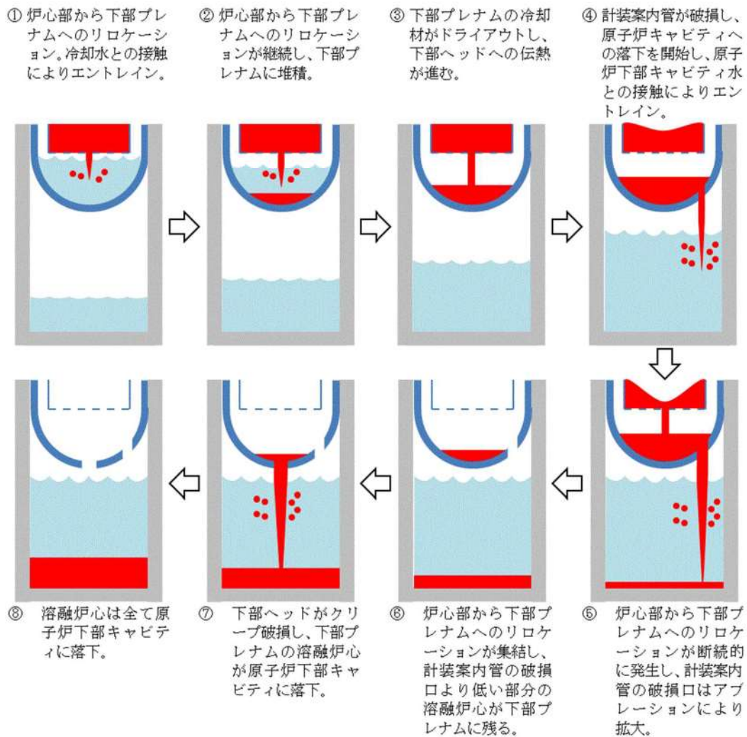
図 3.3-12 原子炉下部キャビティへの熔融炉心の落下の例
