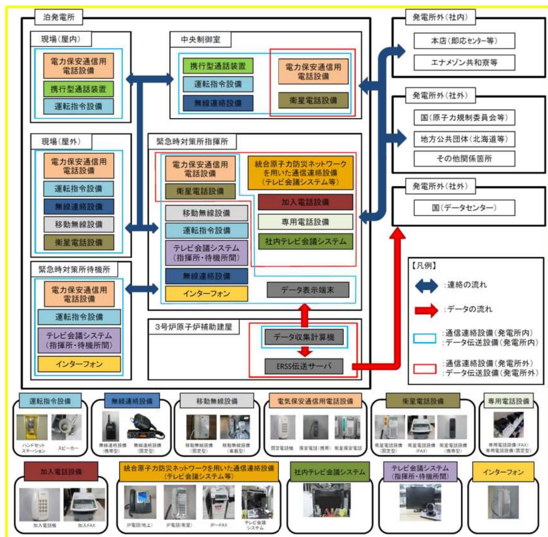
図 2.6-1 緊急時対策所 通信連絡設備の概要
