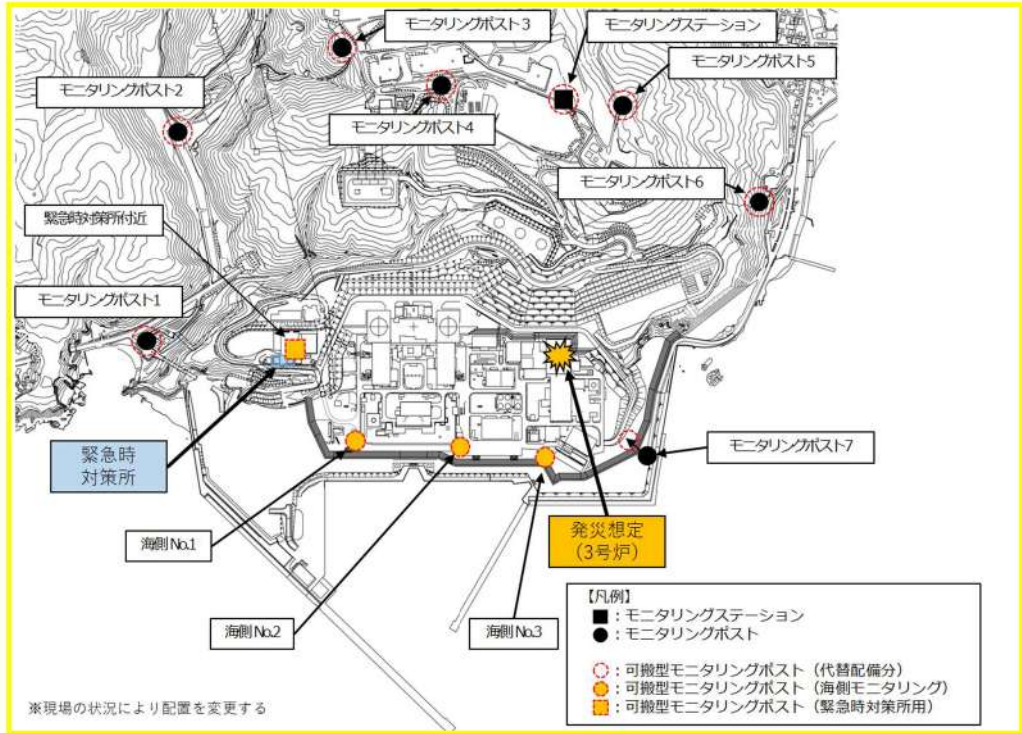
図添 14-2 プルームの状況を検知する手段
