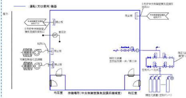
図 2.4-17 5号炉原子炉建屋内緊急時対策所（待機場所）換気設備 系統概略図 （ブルーム通過中：陽圧化装置（空気ポンプ）による陽圧化）
