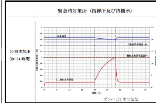
図2.4-9 緊急時対策所指揮所及び緊急時対策所持機所の酸素濃度及び二酸化炭素濃度変化
