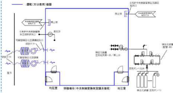
図 2.4-16 5号炉原子炉建屋内緊急時対策所（待機場所）換気設備 系統概略図 （ブルーム通過前及び通過後：可搬型陽圧化空調機による陽圧化）
