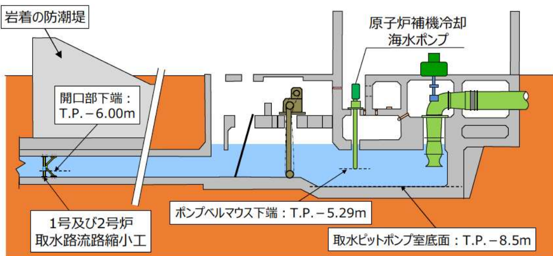
図6 1号及び2号炉取水系 断面（ポンプベルマウス下端）
