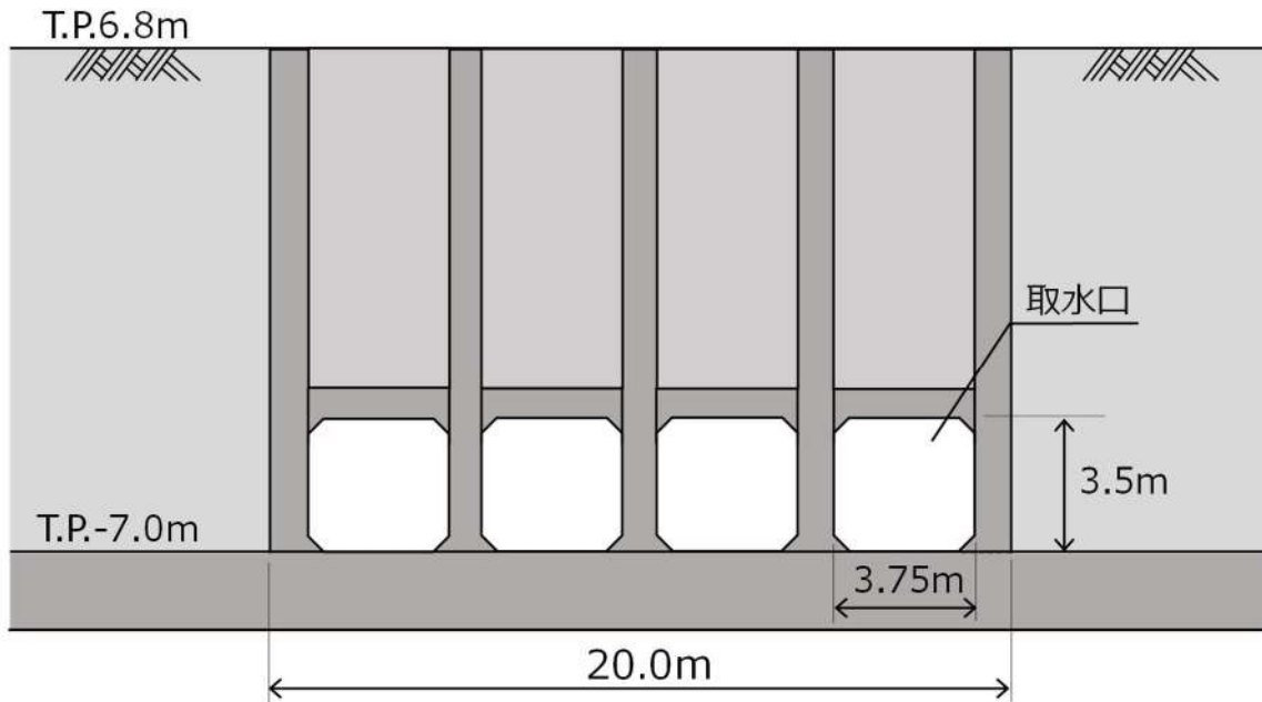
図8 1号及び2号炉取水口概要図
