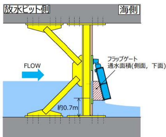
図2 逆流防止設備開口部
