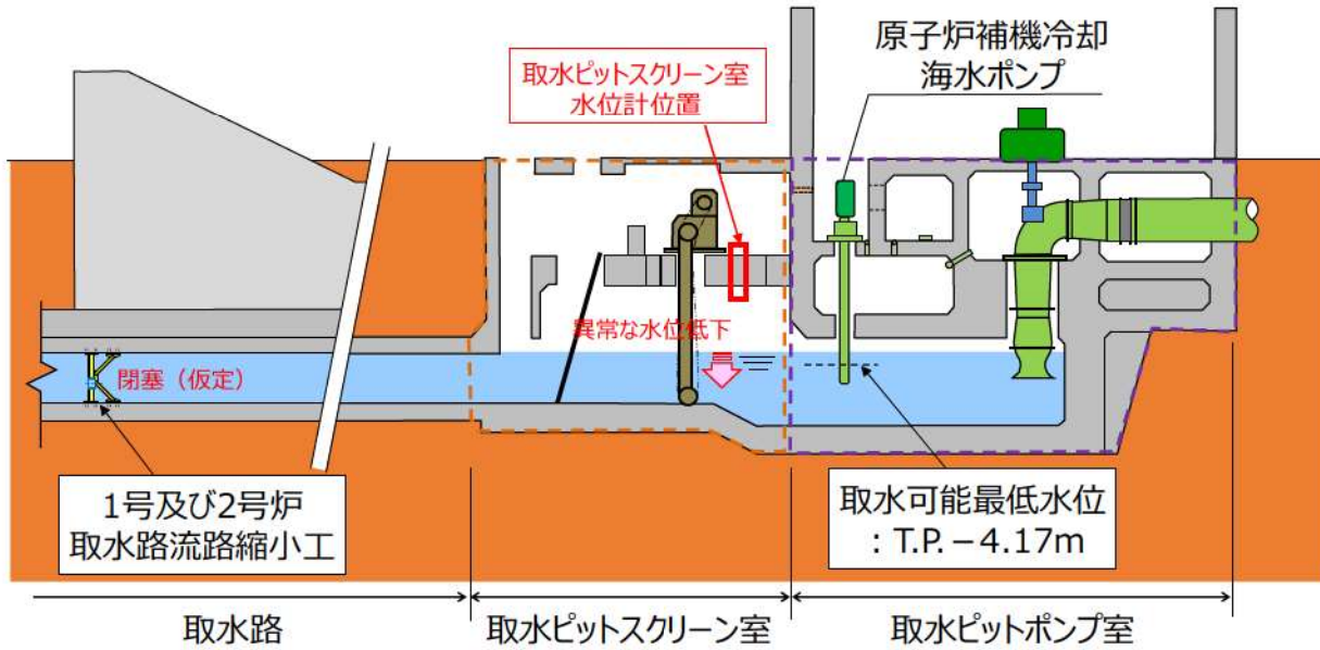
図9 流路縮小工の異常の検知位置
