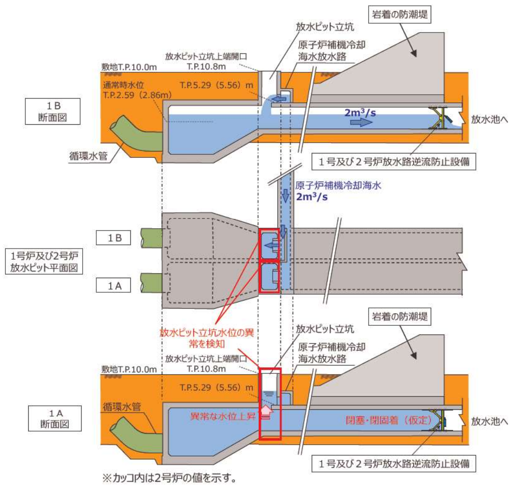
図 8 逆流防止設備の異常の検知位置（1号炉の場合）
