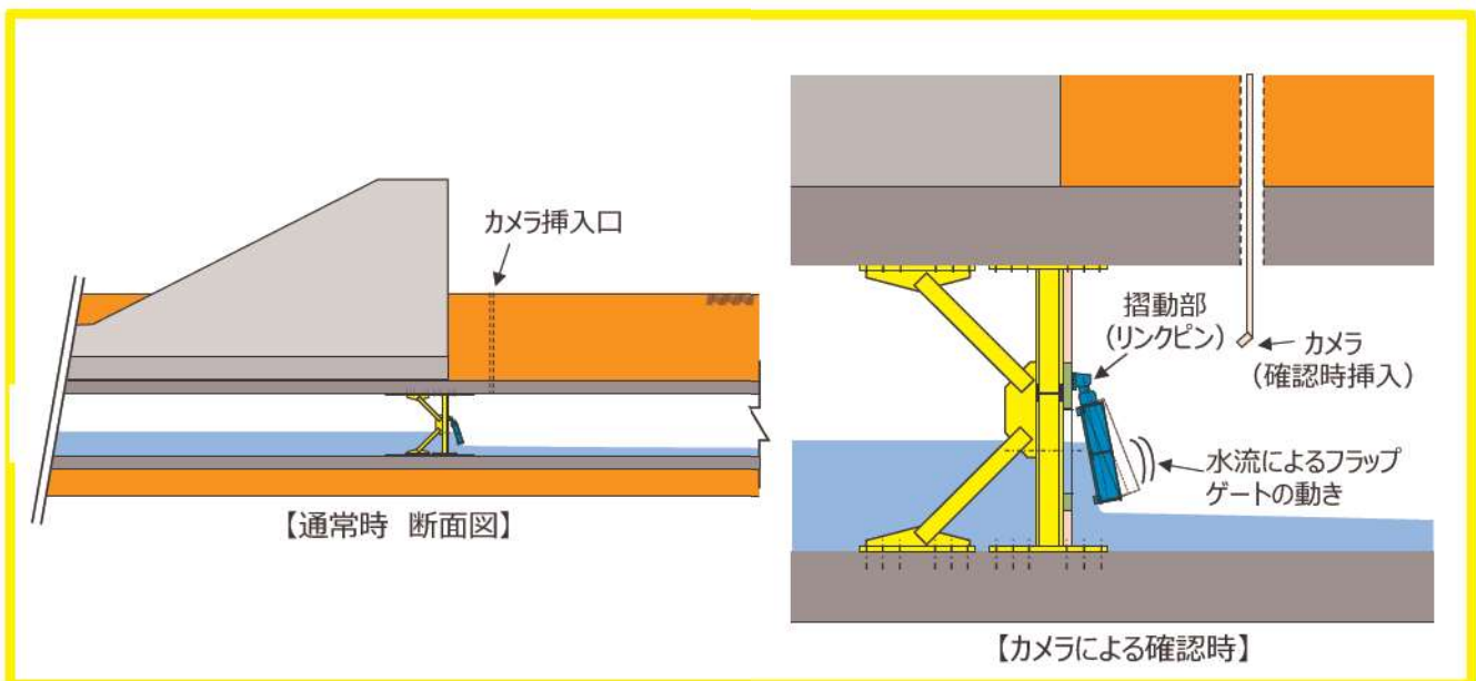
図5 フラップゲートのカメラによる確認のイメージ図
