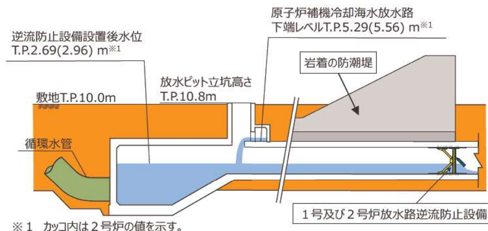
図7 1号及び2号炉放水系断面図
