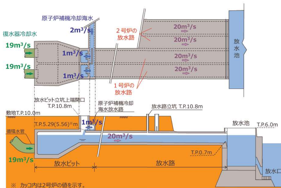
図6 1号及び2号炉放水系概要
