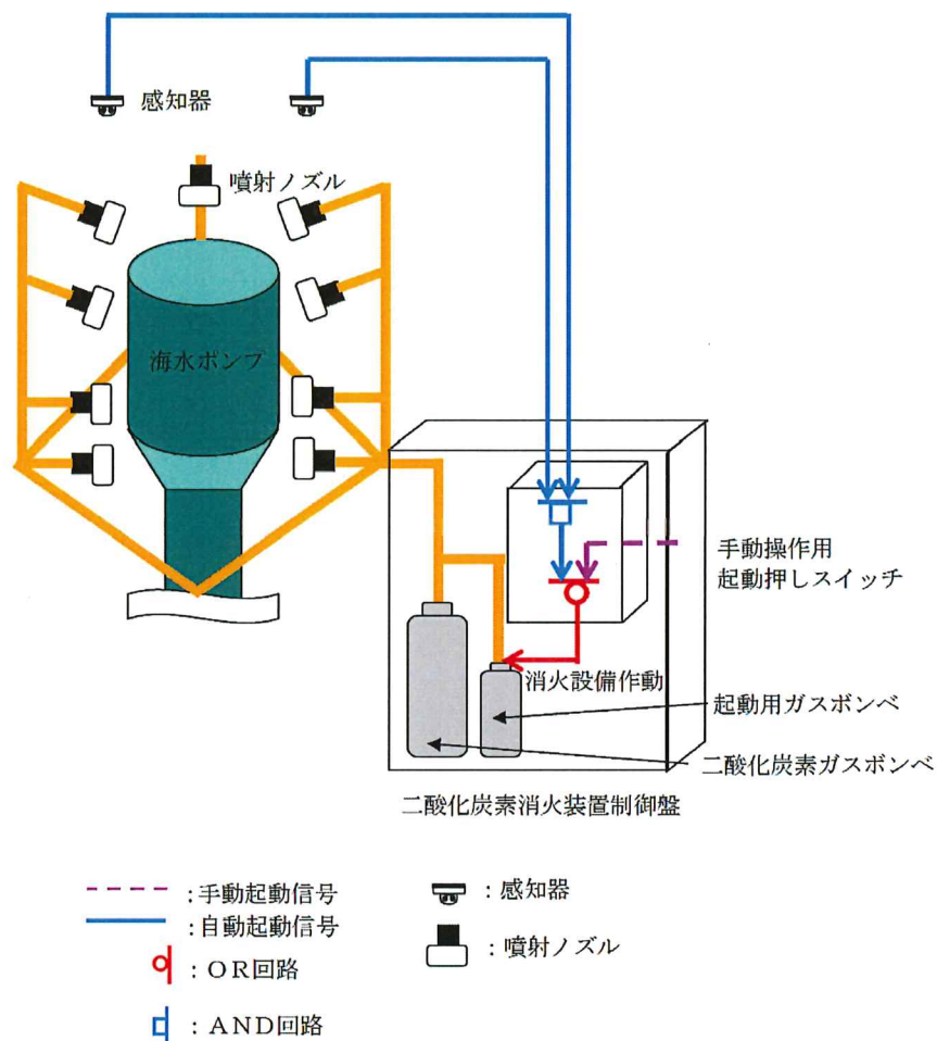
第5-5図 海水ポンプの二酸化炭素消火設備の概要
