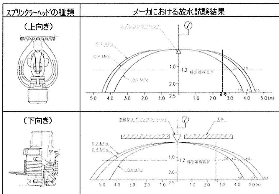
第5-9図 種類別のスプリンクラーヘッドの散水形状
