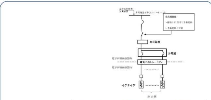
左図：伊方3号、右図：美浜3号の電源構成図を参考掲載
