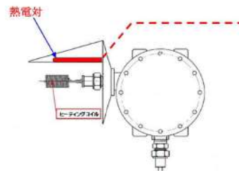
図10 イグナイタへの熱電対取り付け位置
