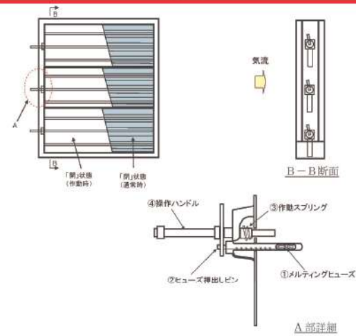
図1-5 ダクト開放機構概略図
