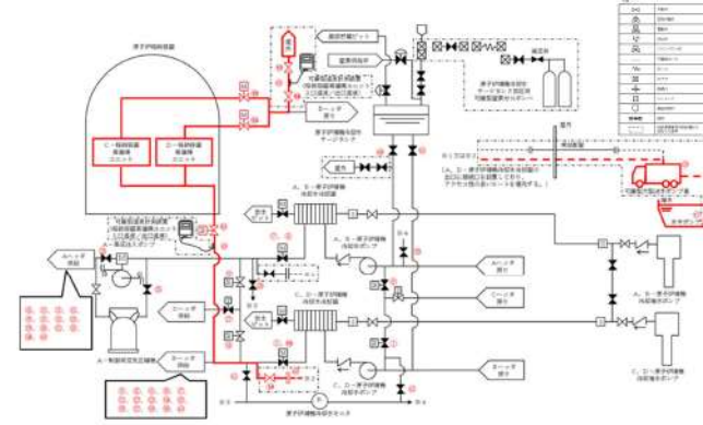
図 49-4-3 格納容器内自然対流冷却
