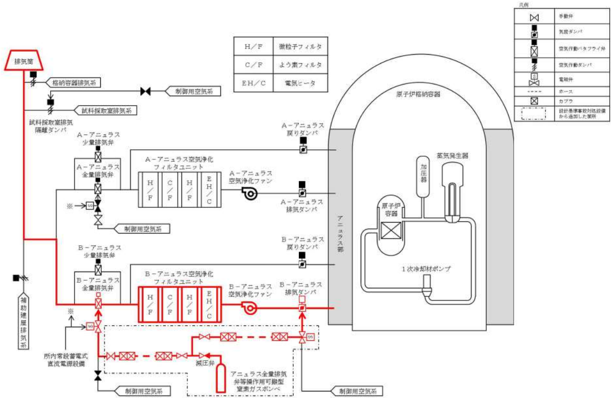
第 53-1 図 アニュラス空気浄化設備による水素排出
