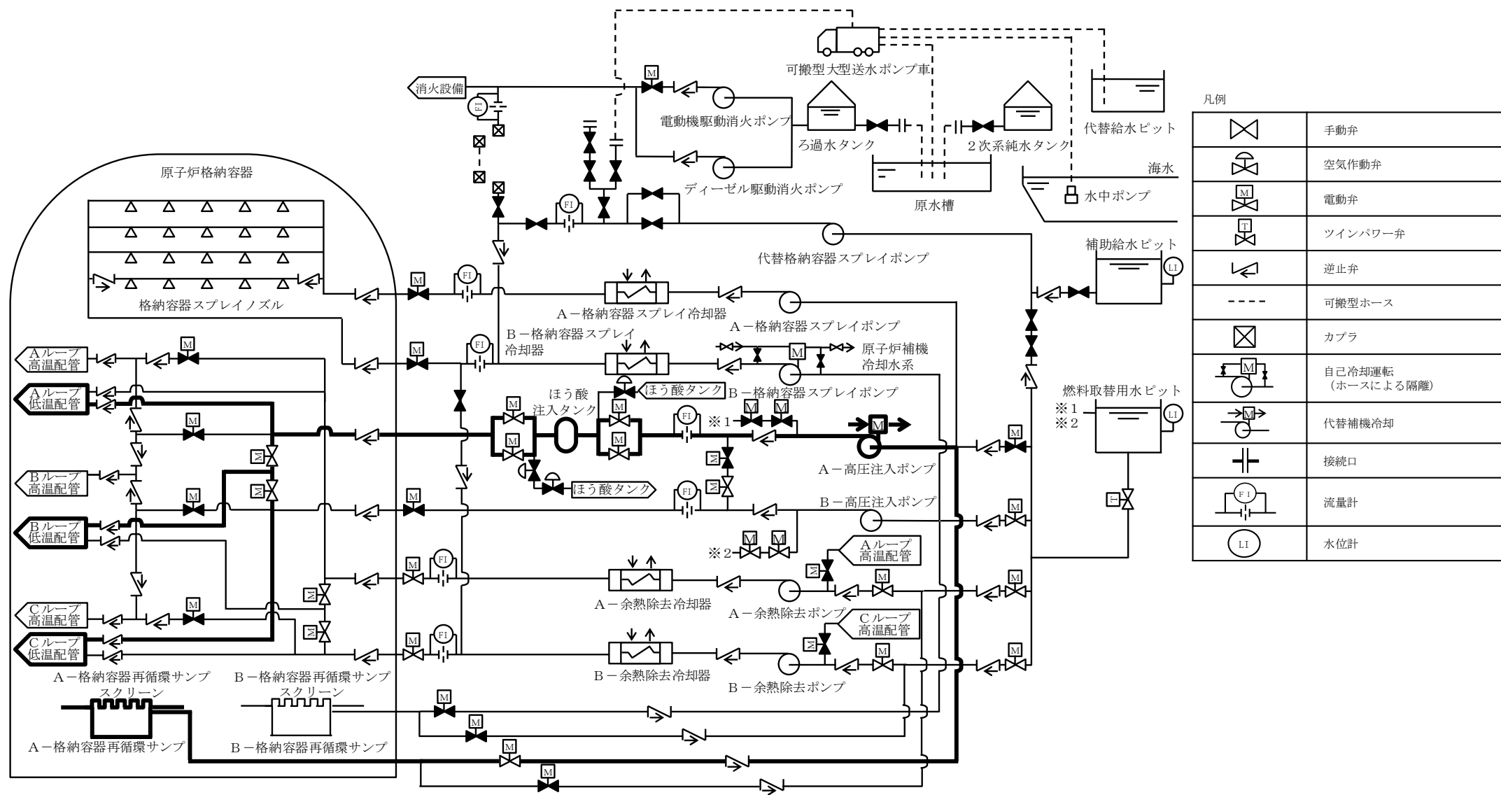
第4.9図 原子炉冷却材圧力バウンダリ低圧時に発電用原子炉を冷却するための設備系統概要図 (7) 代替再循環運転 (A - 高圧注入ポンプ (代替補機冷却) ) [47-51]
