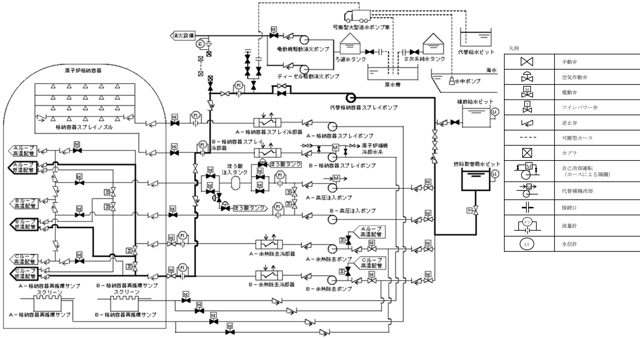
第4.5図 原子炉冷却材圧力バウンダリ低圧時に発電用原子炉を冷却するための設備系統概要図 (3) 代替炉心注水 (代替格納容器スプレイポンプ) [47-47]
