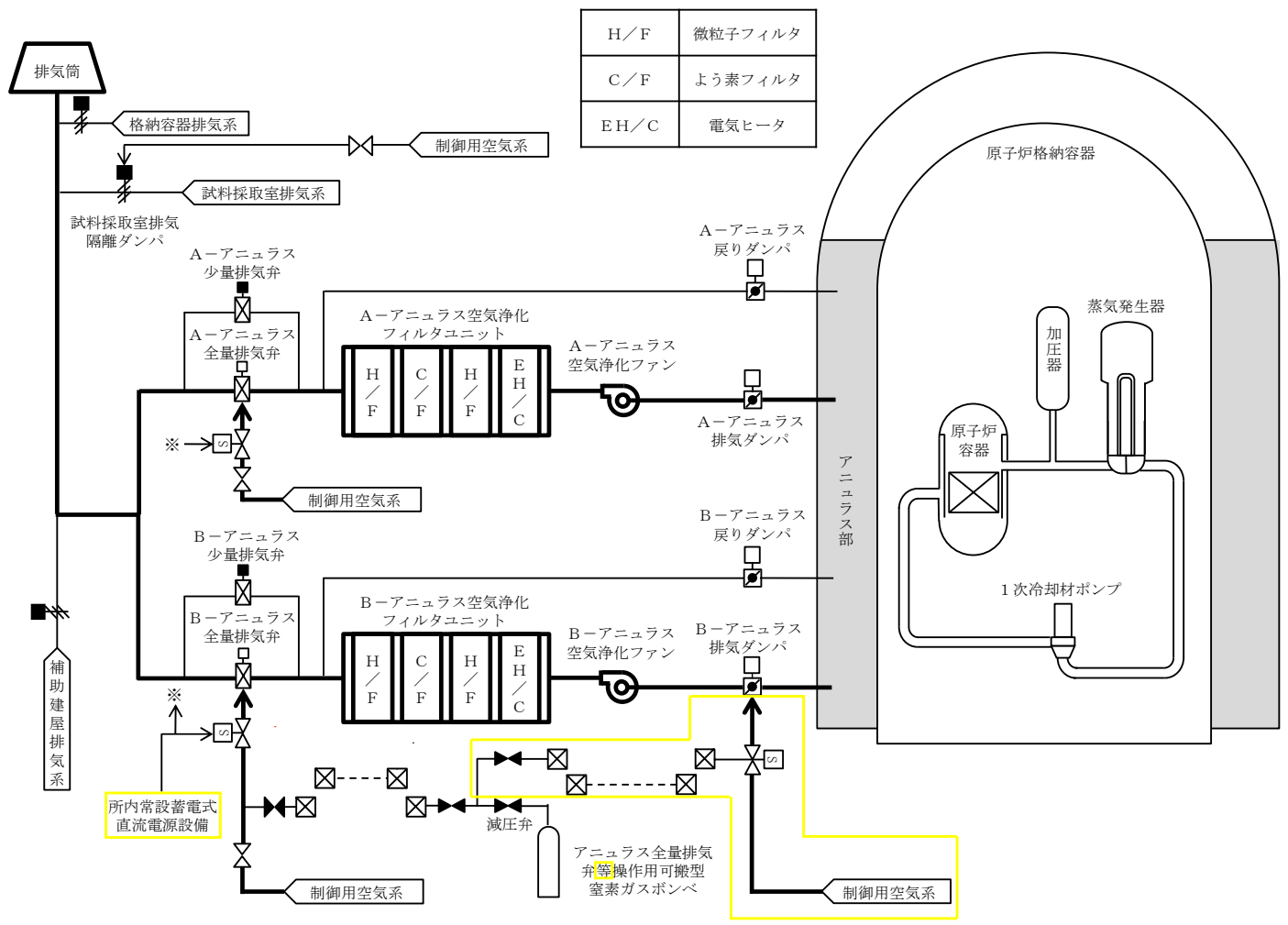
第10.1図 水素爆発による原子炉建屋等の損傷を防止するための設備 系統概要図（1） アニユラス空気浄化設備による水素排出（交流動力電源及び直流電源が健全である場合） [53-14]
