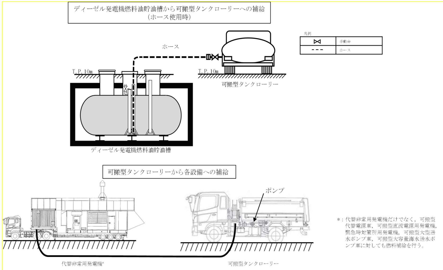
第14.9図 代替電源設備系統概要図 (燃料補給設備による給油) (ディーゼル発電機燃料油貯油槽から各設備への補給 (ホース使用時)) [57-28]
