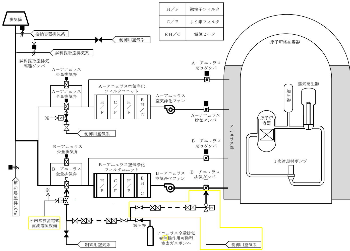
第10.2図 水素爆発による原子炉建屋等の損傷を防止するための設備 系統概要図（2） アニユラス空気浄化設備による水素排出（全交流動力電源又は直流電源が喪失した場合） [53-15]
