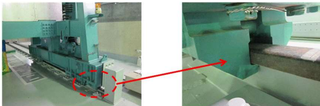
図 5.2.5 転倒防止金具の概要図
