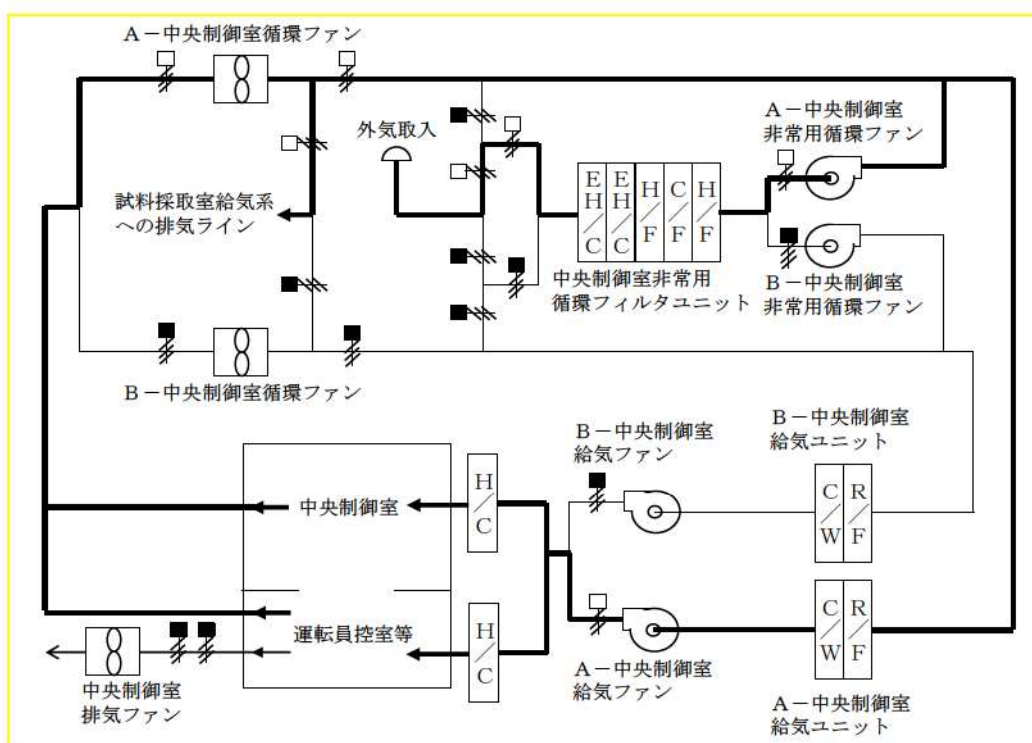
中央制御室空調装置の系統構成概要（外気取入れ運転）
