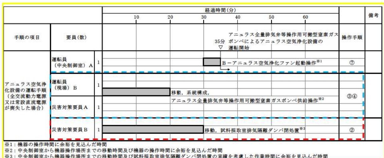
図3 アニオラス空気浄化設備の運転手順 タイムチャート (全交流動力電源又は常設直流電源が喪失した場合)
