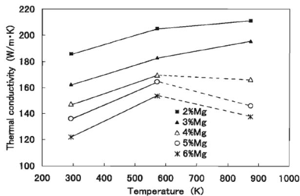
別紙 2-6 図 Al-Mg 合金の熱伝導率と温度の関係に及ぼす Mg 添加量の影響 13)
