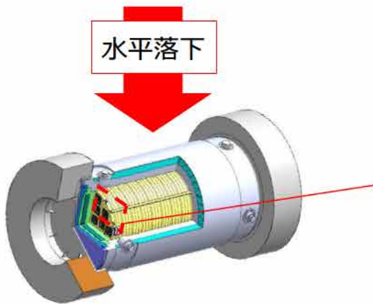
第14図 Hitz-P24 気体マスクのバスケット格子に引張応力の発生が予想されるケース
