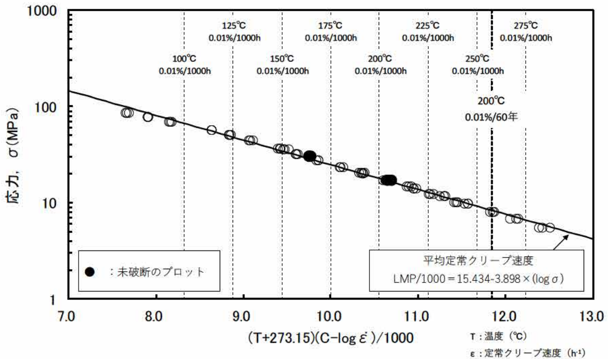
第 7-32 図 応力-定常クリーブ速度プロット
