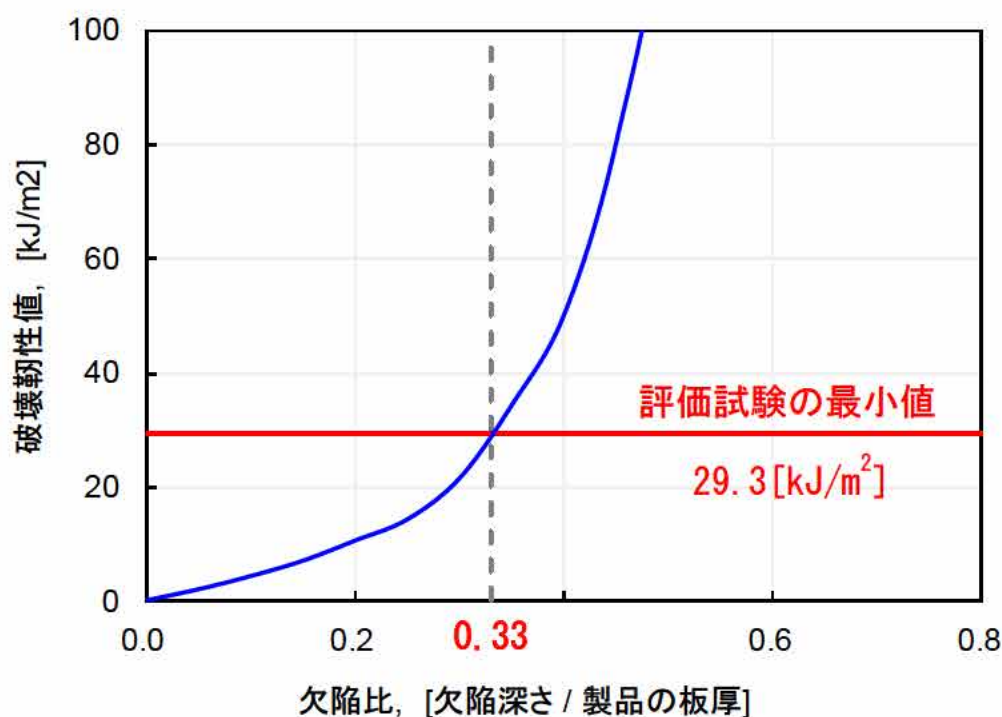
第16図 欠陥比と破壊靱性値の関係
