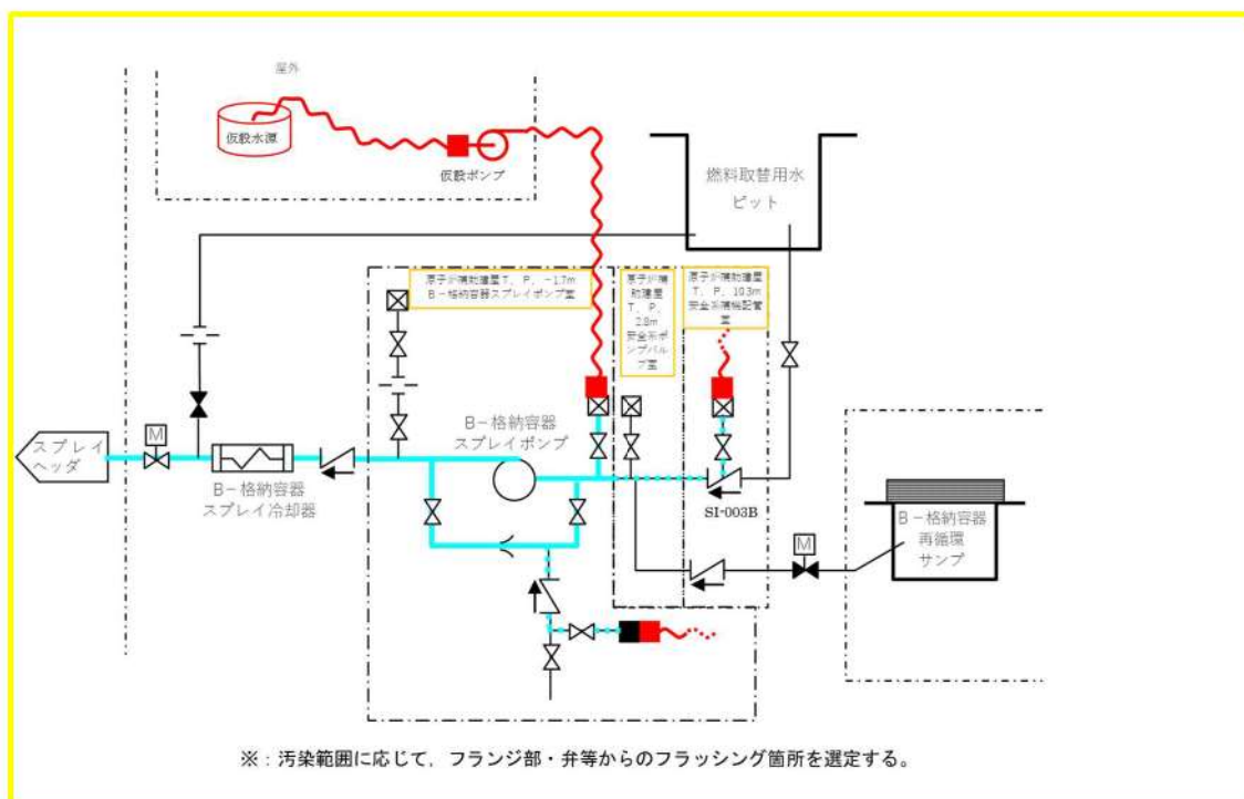
図5 格納容器スプレイラインのフラッシング概要図
