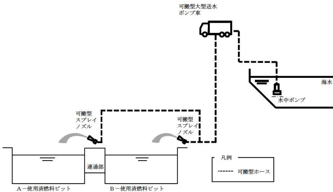
図2 海水を用いた可搬型大型送水ポンプ車及び可搬型スプレィノズルによる泊1, 2号炉 SFP へのスプレィ 概略系統
