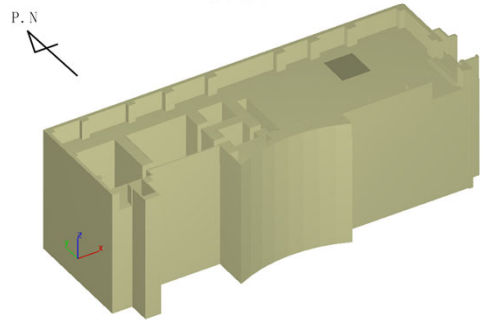
図8-1 使用済燃料ピット周辺の機器配置図及び解析モデル図
