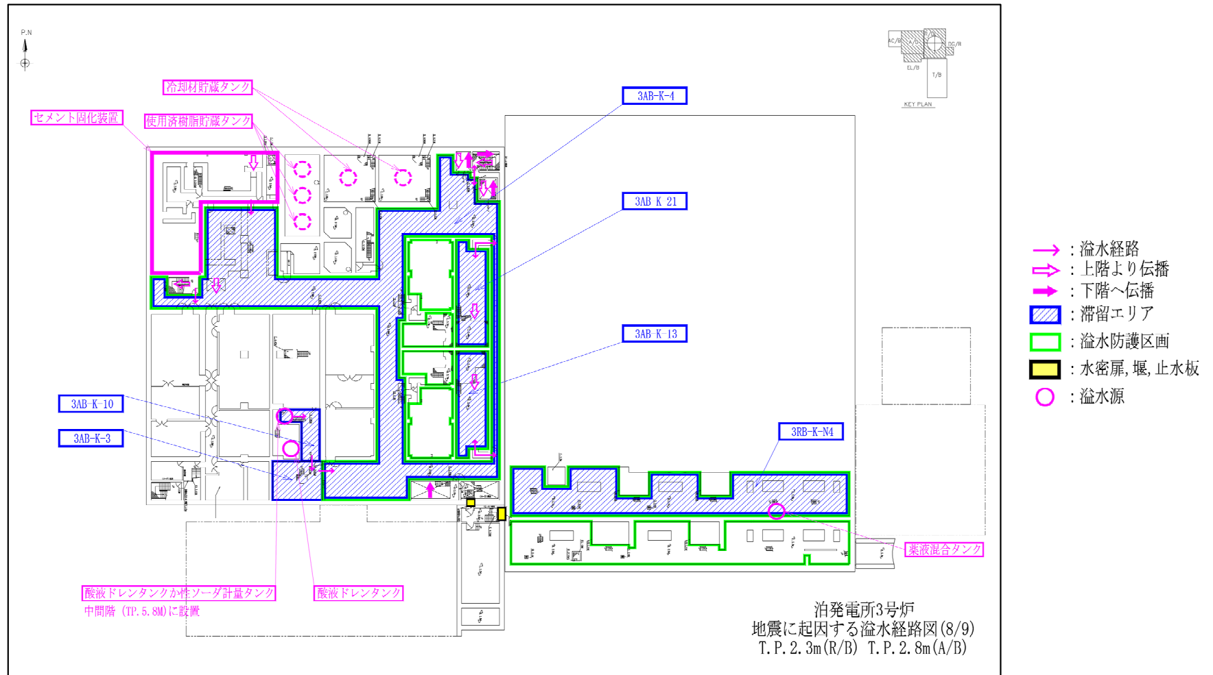
図4-2 地震に起因する溢水経路図
