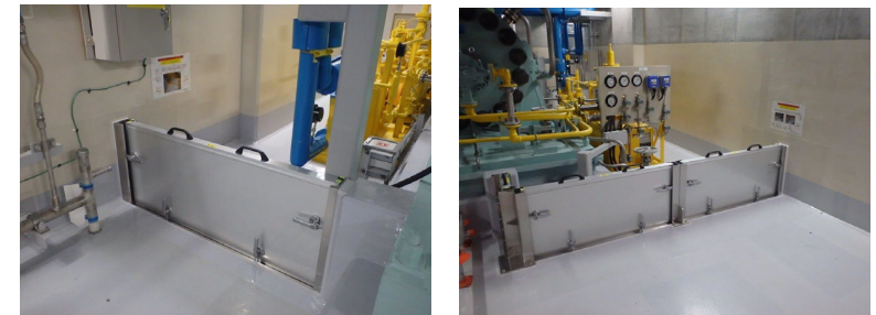
図5-4 止水板設置状況
