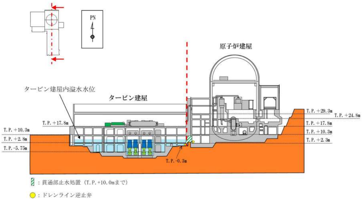
図 9-1 タービン建屋断面図
