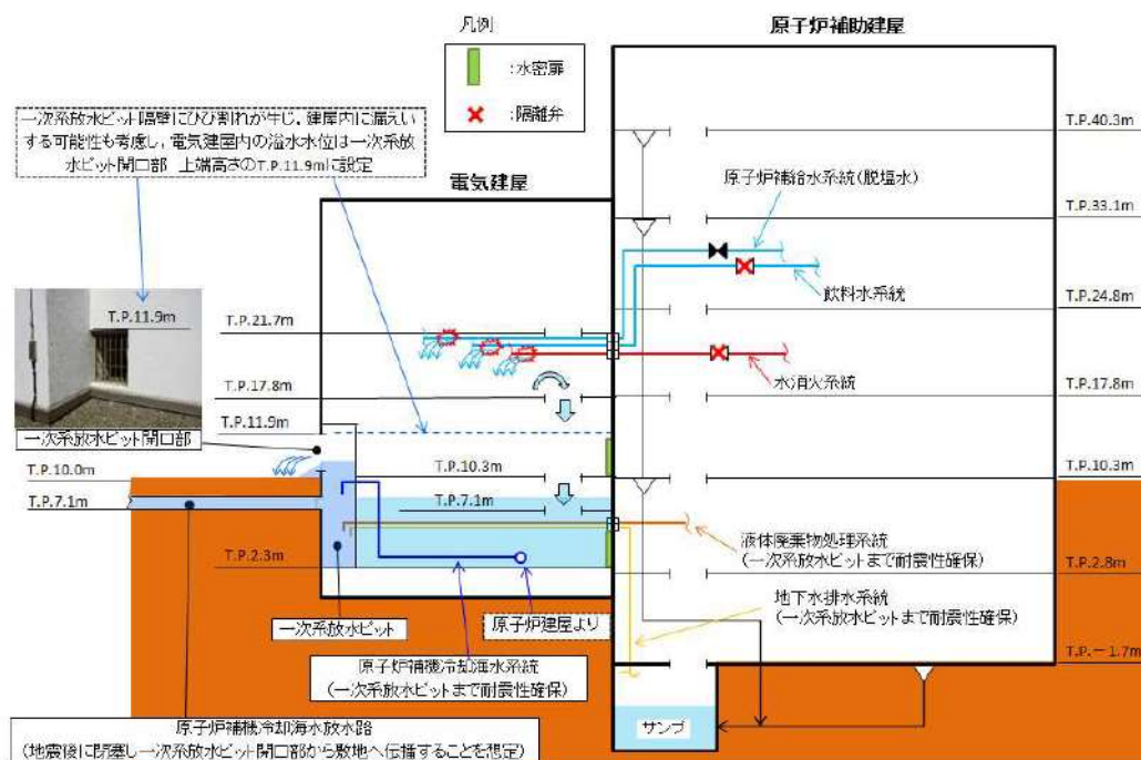
図 10-1 電気建屋の溢水概念図
