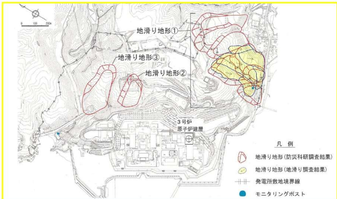
第 1.12.1-1 図 泊発電所周辺の地滑り地形位置図
