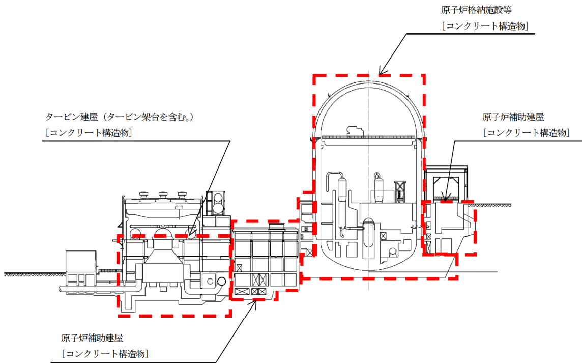
原子炉格納施設等・原子炉補助建屋・タービン建屋 [コンクリート構造物]
