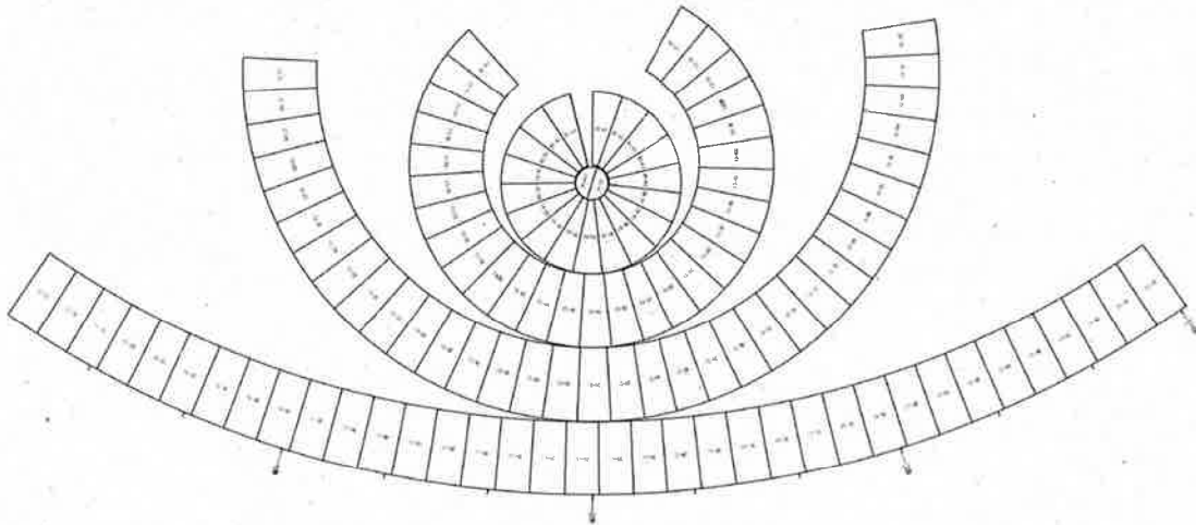
板割図 (半球部 内面)
