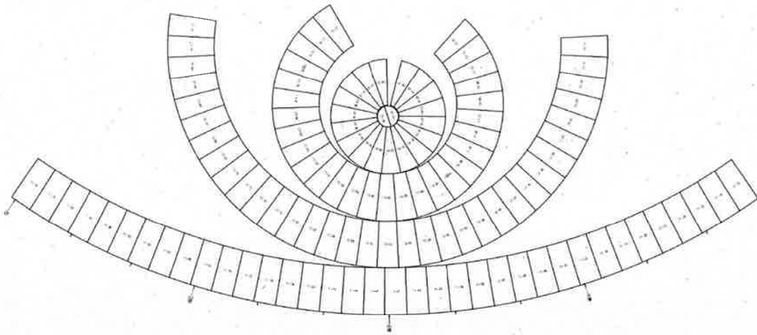
板割図 (半球部 外面)
