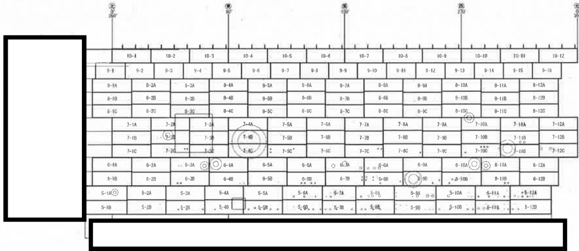
板割図 (円筒部 内面)
