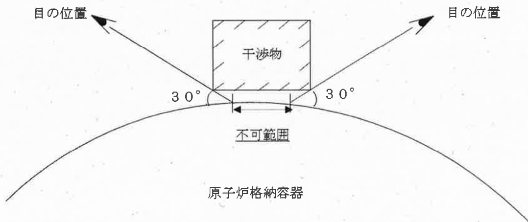
図4-1 干渉物が単独で存在する場合
