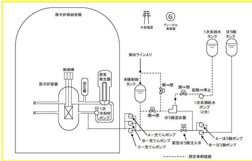
図1 「原子炉起動時に、化学体積制御系の弁の誤動作等により原子炉へ純水が流入する事故」の重大事故等対策の概略系統図 (希釈停止操作)
