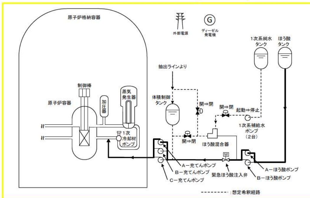
図2 「原子炉起動時に、化学体積制御系の弁の誤動作等により原子炉へ純水が流入する事故」の重大事故等対策の概略系統図 (ほう酸注入)
