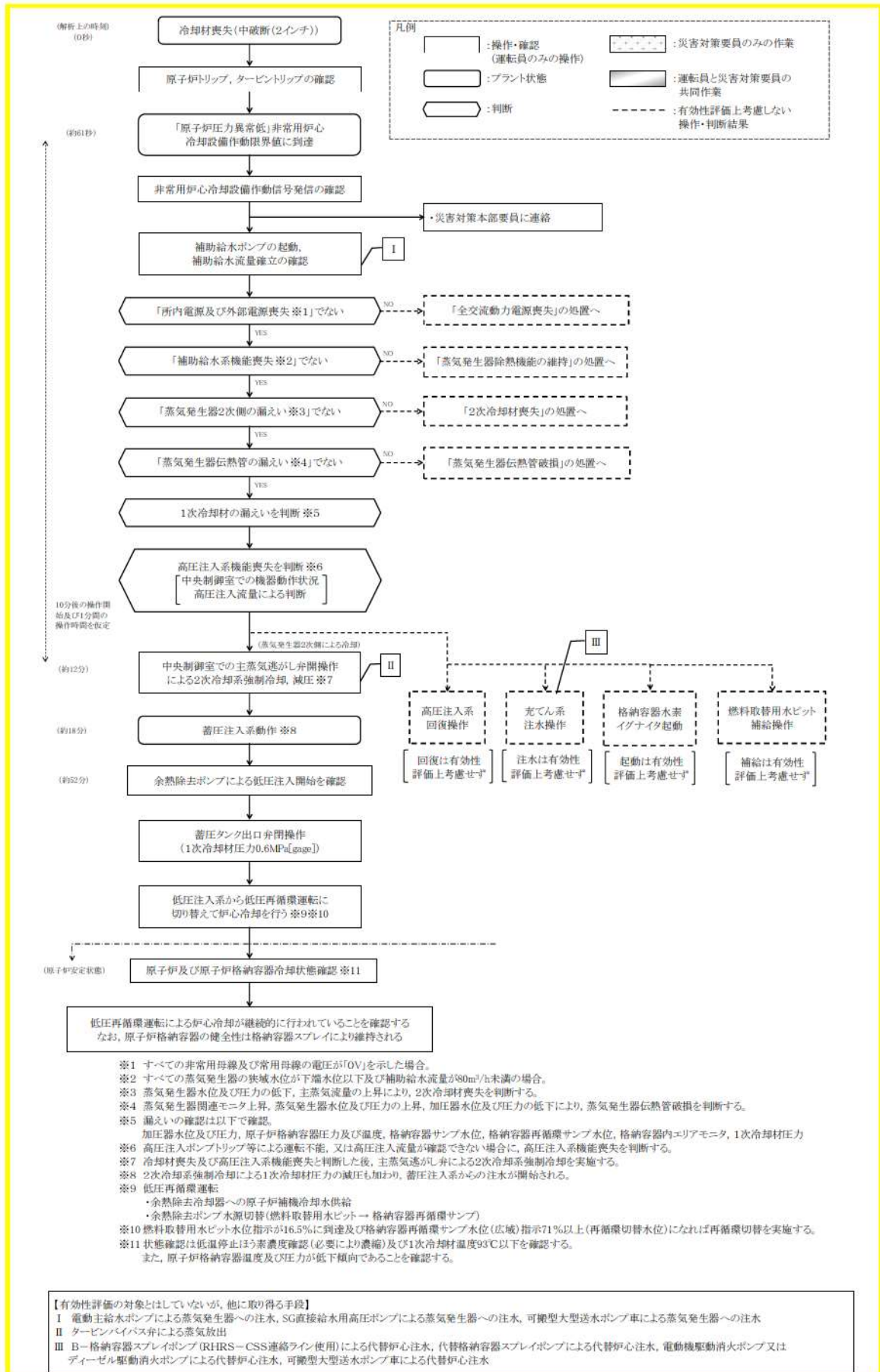
第 7.1.6.5 図 「ECCS 注水機能喪失」の対応手順の概要 (「中破断 LOCA (2 インチ破断) 時に高圧注入機能が喪失する事故」の事象進展)
