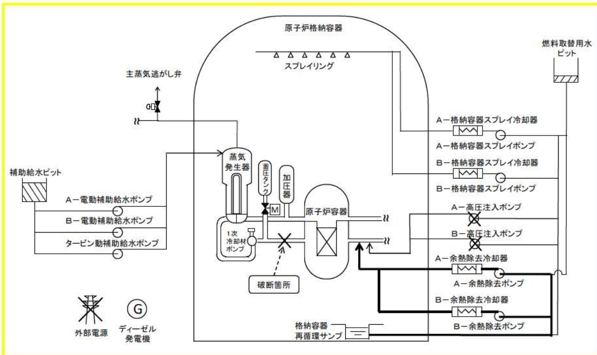
図2 「中破断 LOCA 時に高圧注入機能が喪失する事故」の重大事故等対策の概略系統図（低圧再循環）
