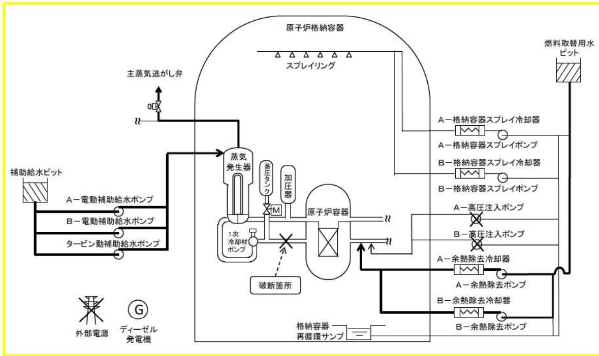
図1 「中破断 LOCA 時に高圧注入機能が喪失する事故」の重大事故等対策の概略系統図（2次冷却系強制冷却及び低圧注入）
