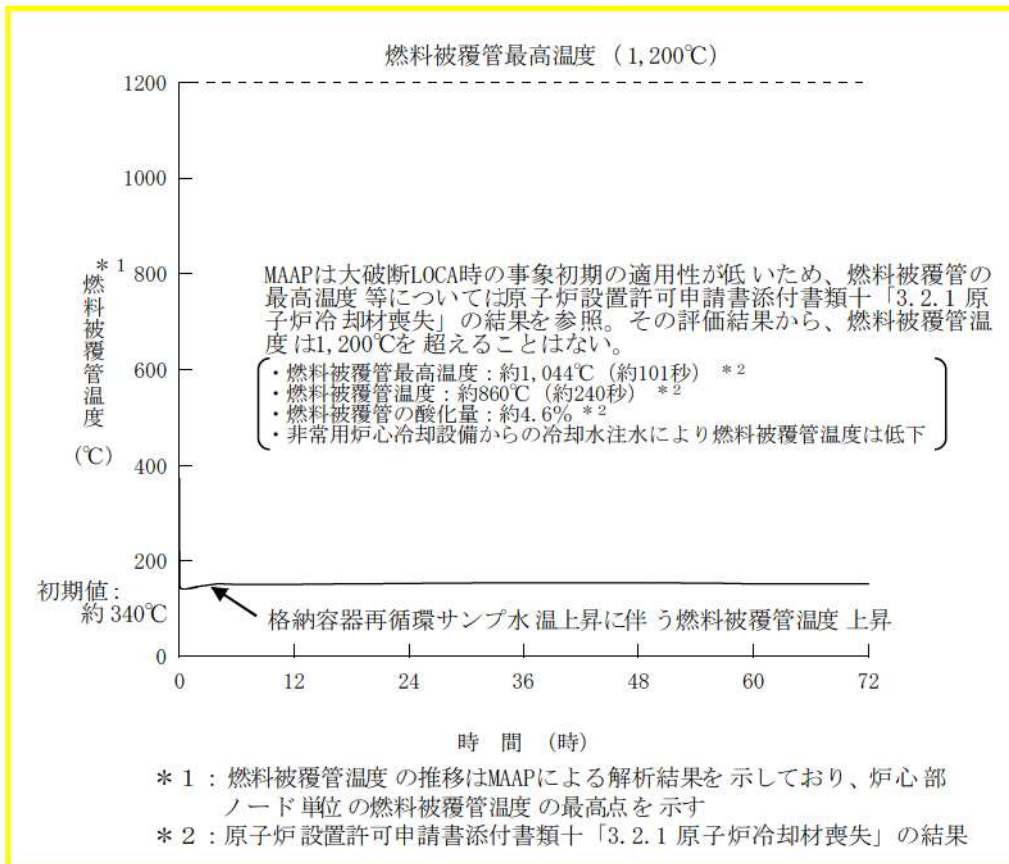
第 7.1.4.10 図 燃料被覆管温度の推移
