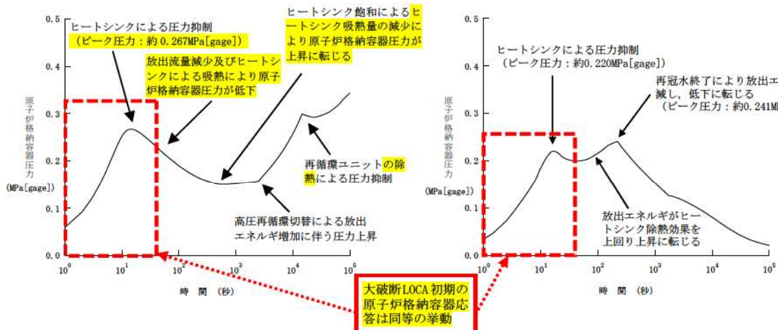
(a) 大破断 LOCA 時に低圧再循環機能及び格納容器スプレイ注入機能が喪失する事故 (MAAP) (b) 原子炉冷却材喪失 原子炉格納容器健全性評価用内圧解析 (SATAN-VI/WREFLOOD/COCO)
