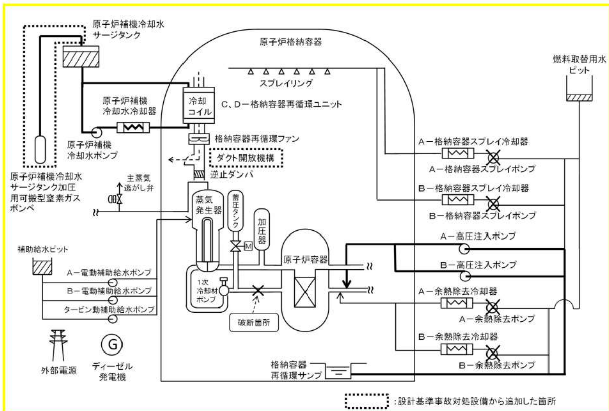
第 7.1.4.1 図 「原子炉格納容器の除熱機能喪失」の重大事故等対策の概略系統図 (2/2) (高圧再循環及び格納容器内自然対流冷却)
