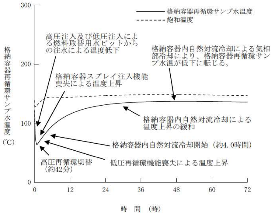
第 7.1.4.12 図 格納容器再循環サンプ水温度の推移
