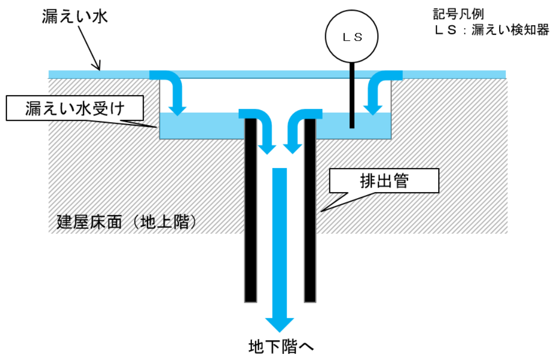
図－1 堰内排出口概念図
