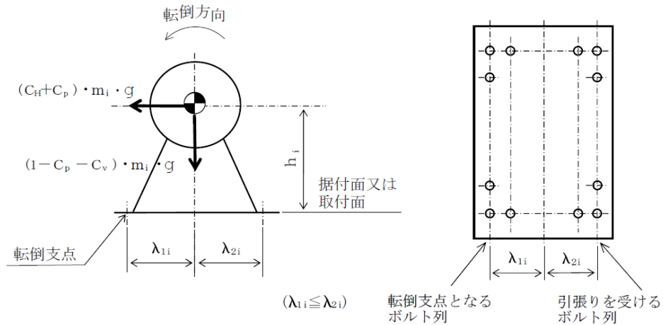
図3-1 計算モデル (軸直角方向転倒の場合)
