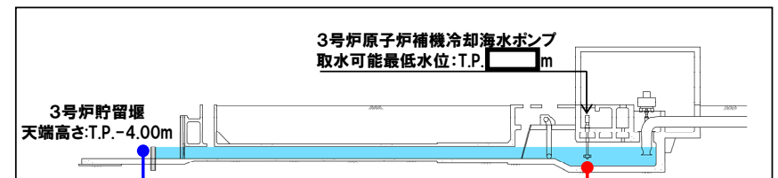
《3号炉貯留堰～取水路、取水ピット縦断面図》
