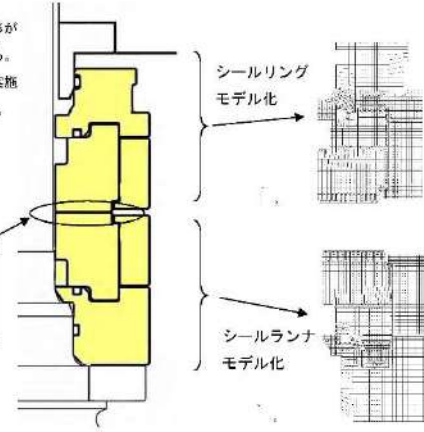
図3 No. 1シールの変形解析モデル
