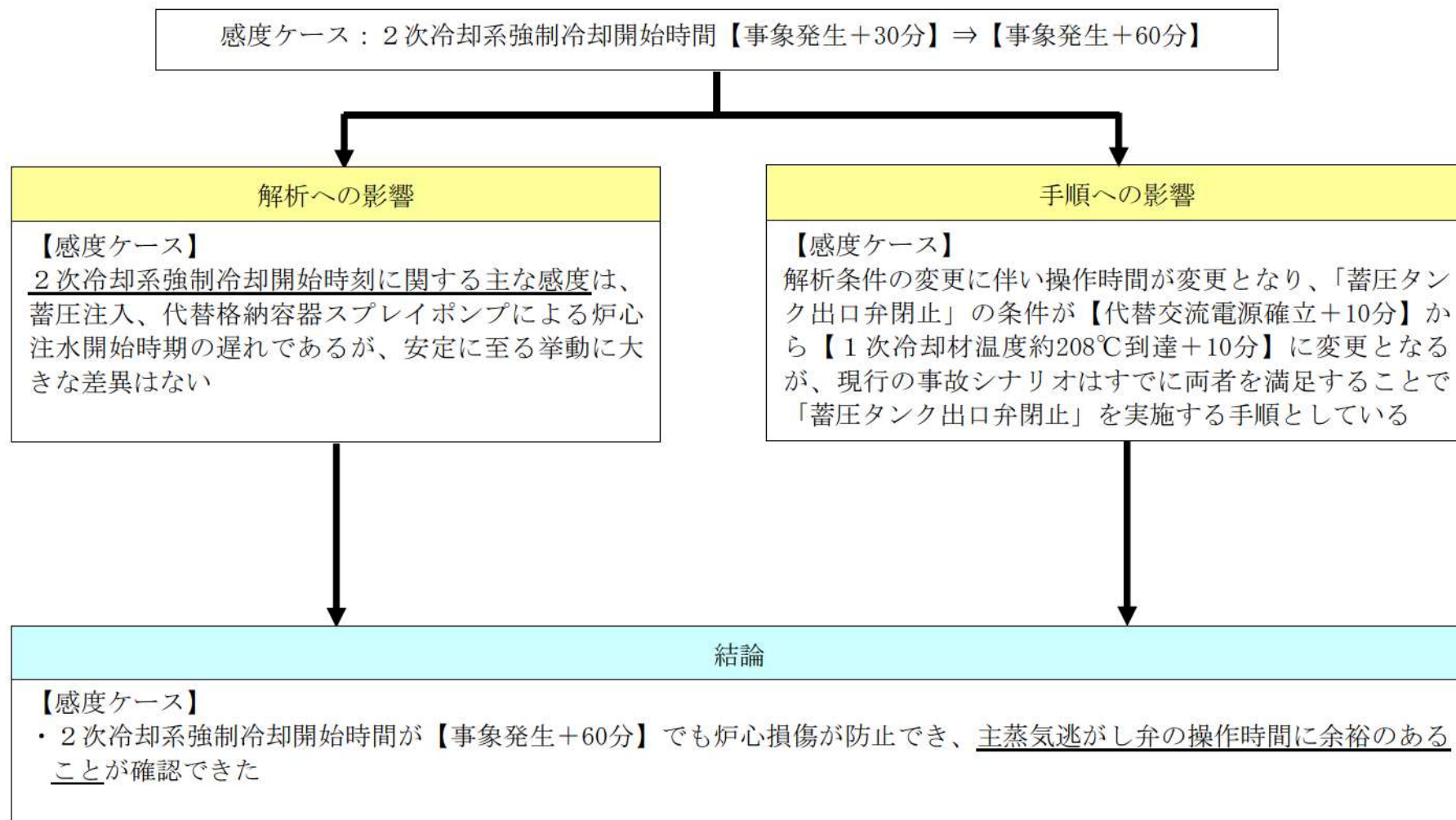
図5 感度ケースの解析、手順への影響確認結果
