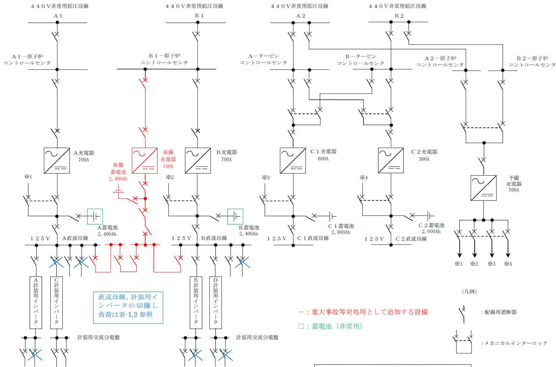
図-1 直流電源単線結線図
