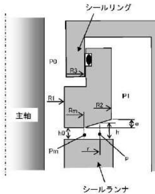
図4 計算モデル
