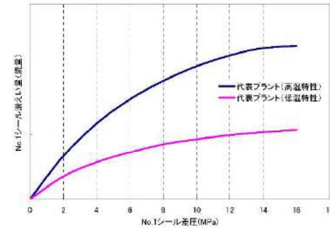
図5 No. 1シールの差圧と漏えい量の関係
