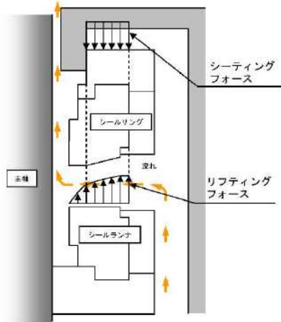
図1 No. 1シールの作動原理模式図
