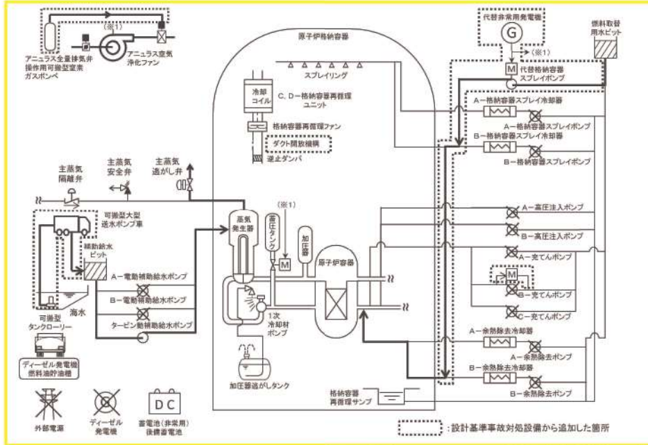
図1 「外部電源喪失時に非常用所内交流電源が喪失し、原子炉補機冷却機能の喪失及びRCPシールLOCAが発生する事故」の重大事故等対策の概略系統図 (2次冷却系強制冷却及び代替炉心注水)
