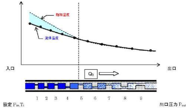
図1 計算モデル
