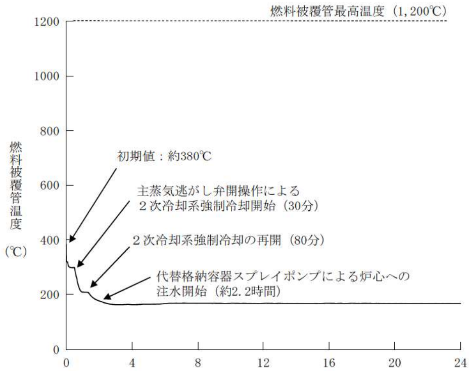
第 7. 1. 2. 17 図 燃料被覆管温度の推移 (RCP シール LOCA が発生する場合)
