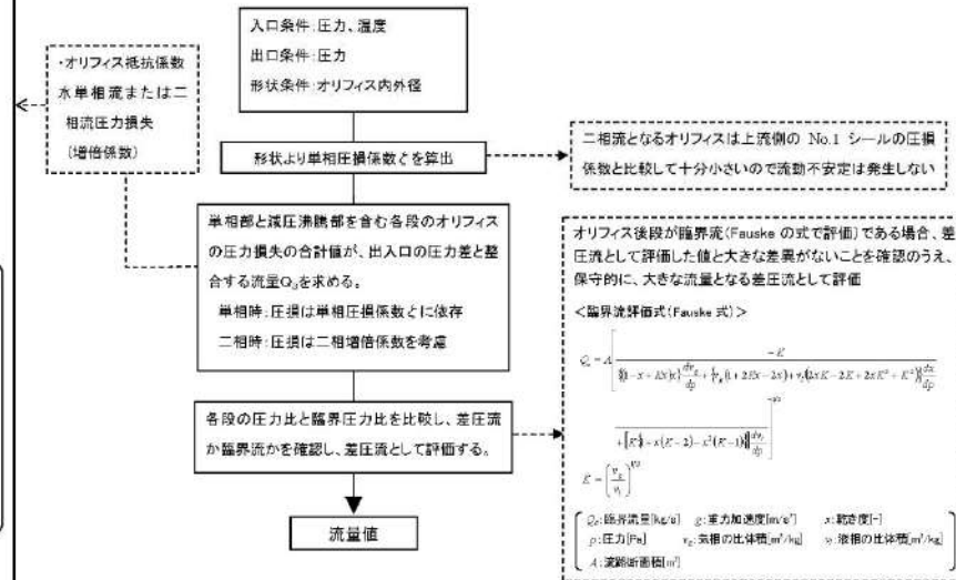
図2 計算フロー
