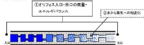
図2 計算モデルの考え方(オリフィス)
