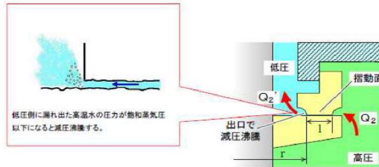
図1 計算モデル
