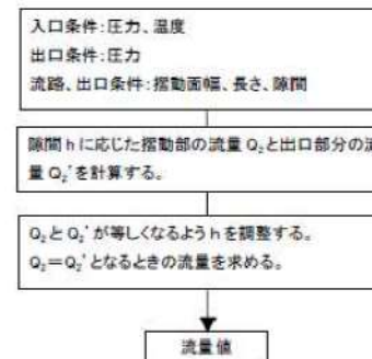
図2 計算フロー
