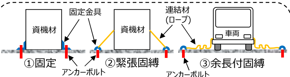
図9 飛来物発生防止対策（固定及び固縛）の例
