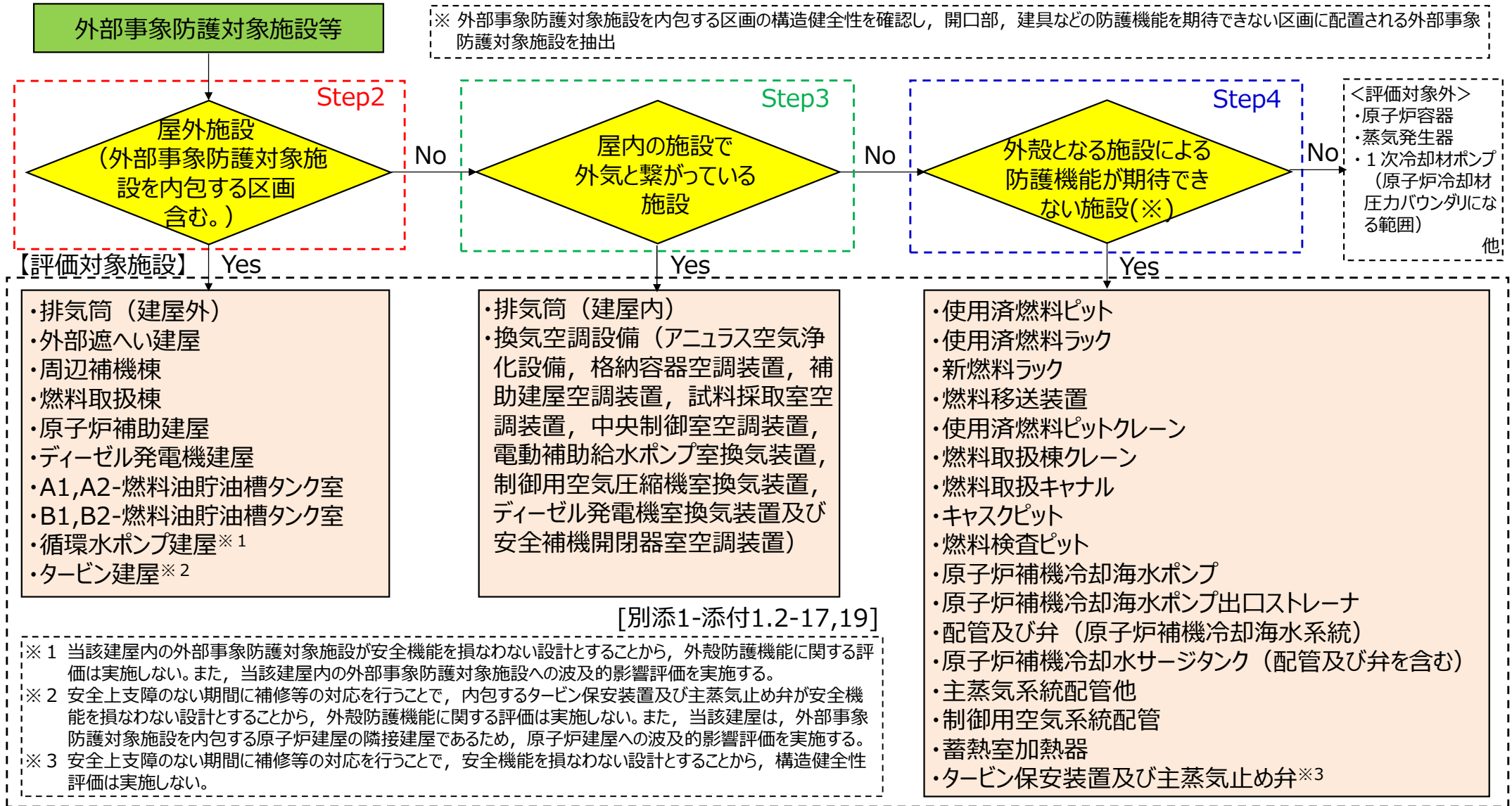
第1.2.2.2図 外部事象防護対象施設等のうち評価対象施設の抽出フロー
