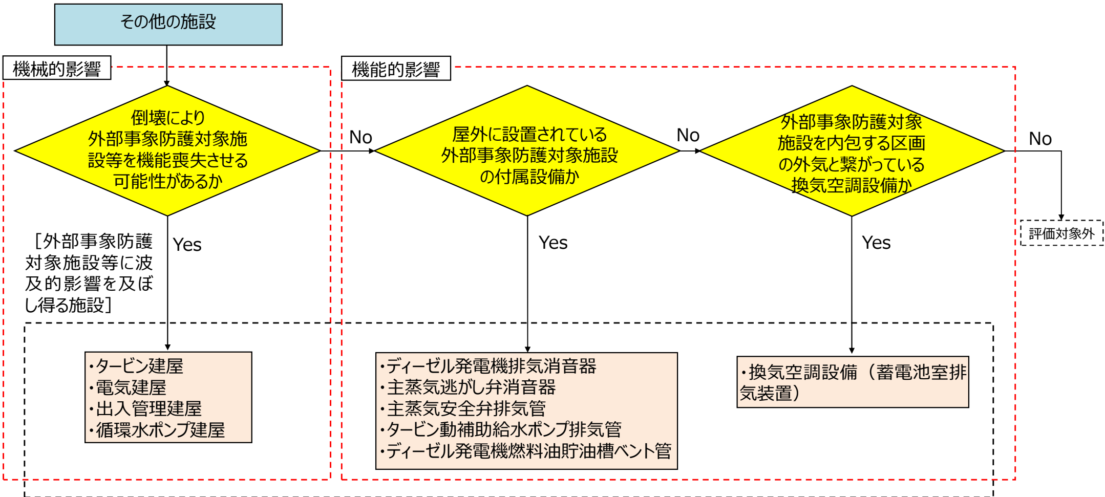
第1.2.2.4図 外部事象防護対象等に波及的影響を及ぼし得る施設の抽出フロー
