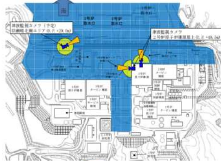
図2.1-4 2号炉原子炉棟と津波監視カメラの監視可能な範囲
