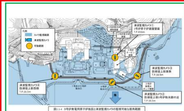
図2.1-4 3号炉原子炉棟と津波監視カメラの監視可能な範囲
