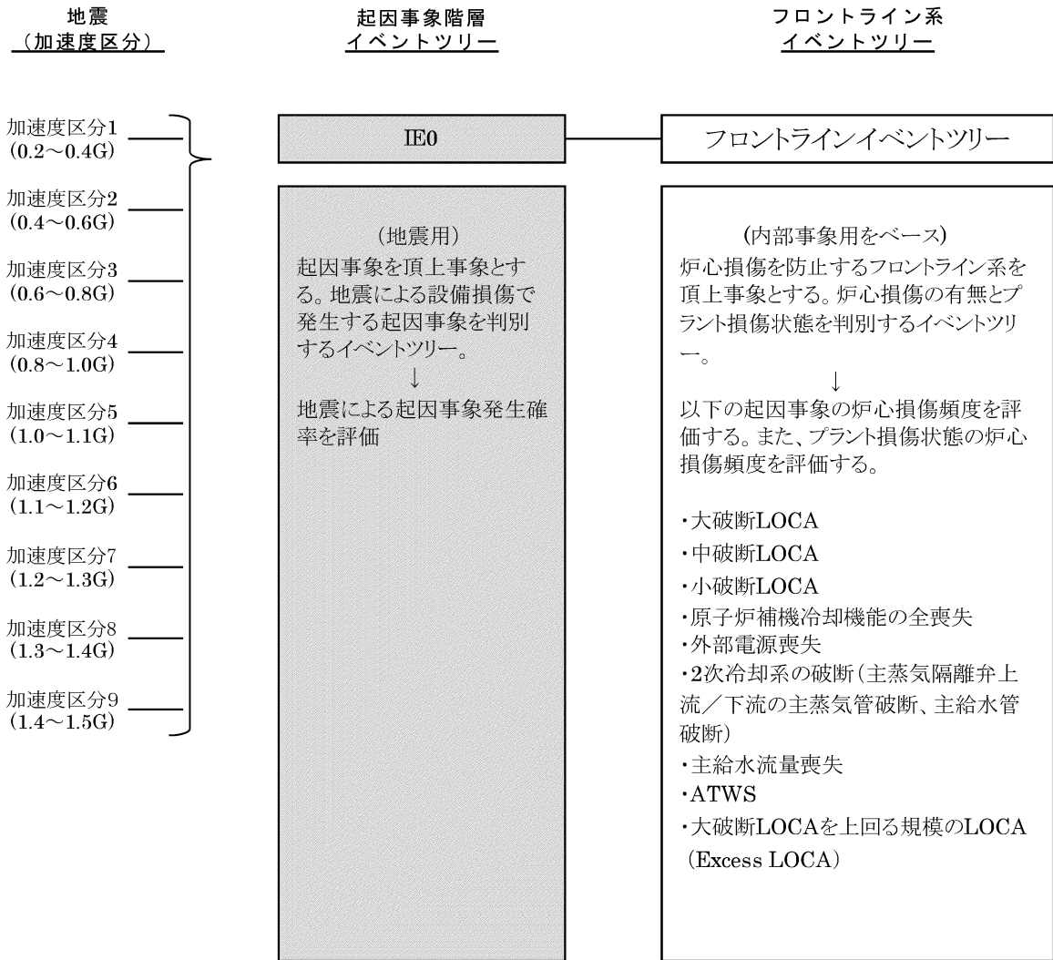
第 3.1.3.2.1.4.1 図 地震システム解析モデル
