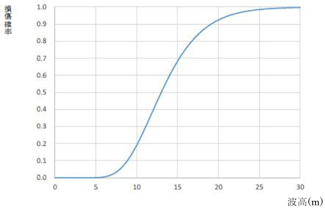
第 3.1.3.2.2.3.4 図 フラジリティ曲線（被水・没水（屋外）：設置 E.L.13.0m）
