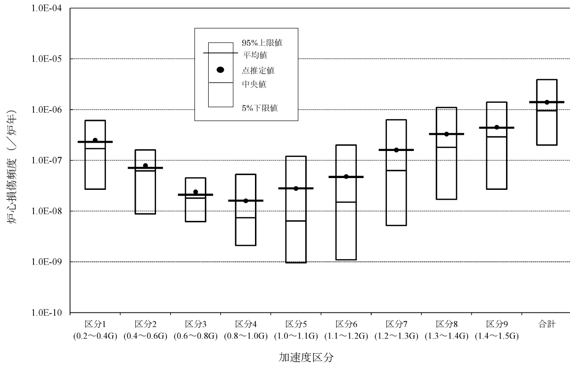
第 3.1.3.2.1.4.16 図 炉心損傷頻度の不確実さ解析結果
