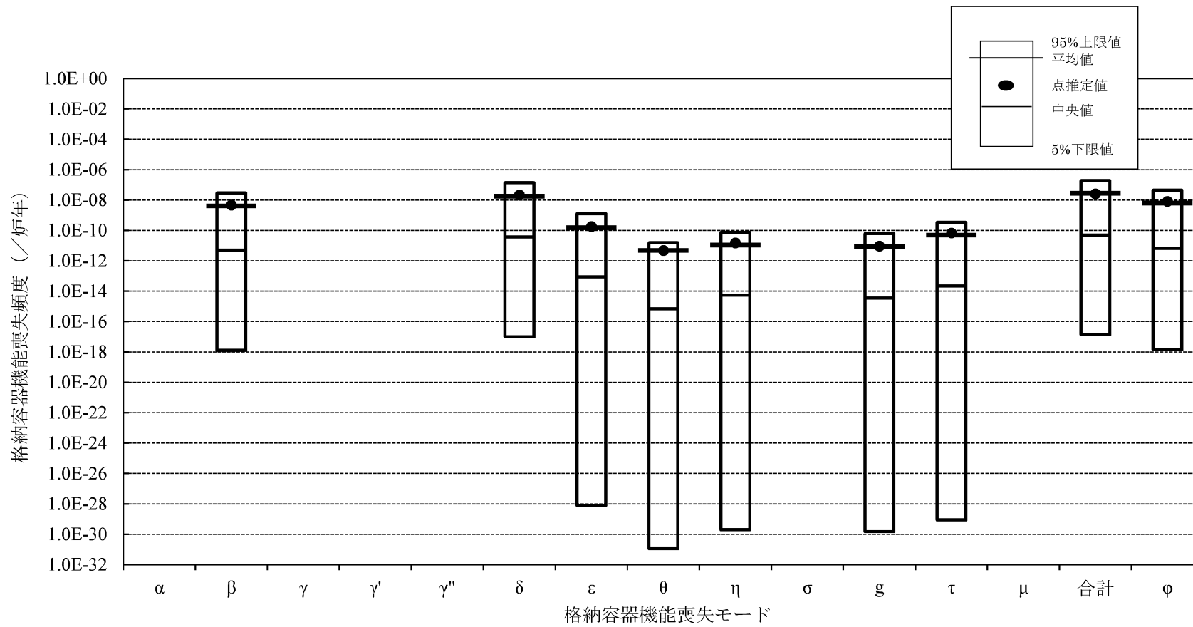
第 3.1.3.2.2.5.3 図 格納容器機能喪失頻度の不確実さ解析結果 (格納容器機能喪失モード別)
