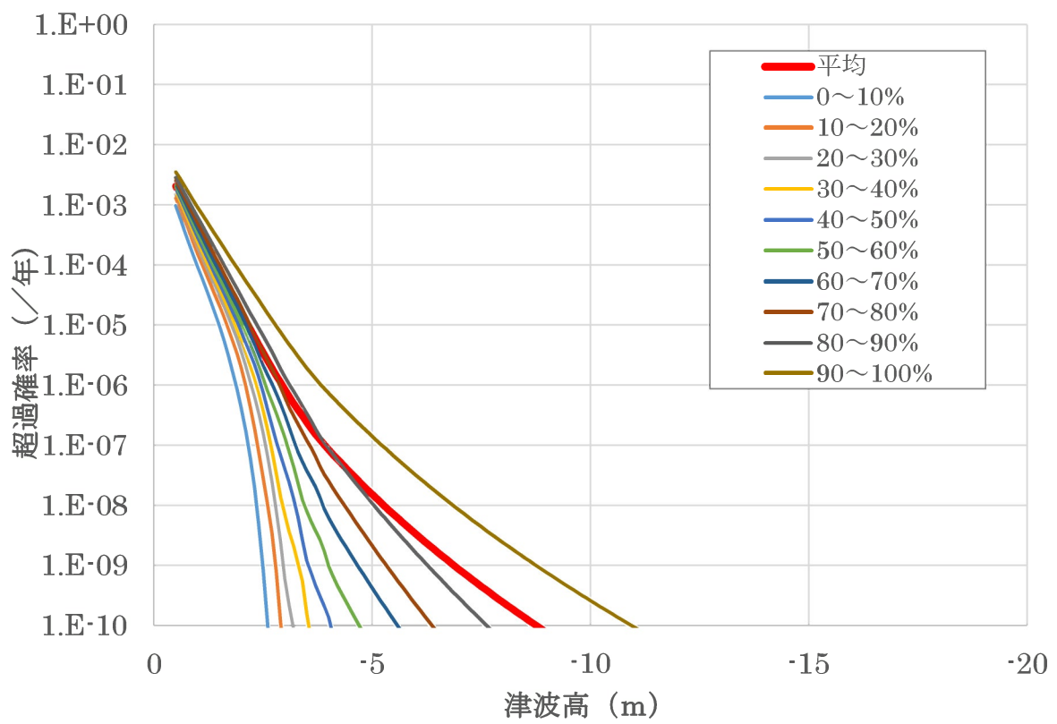
第 3.1.3.2.2.19 図 フラクタル津波ハザード曲線 (上：水位上昇側、下：水位下降側)
