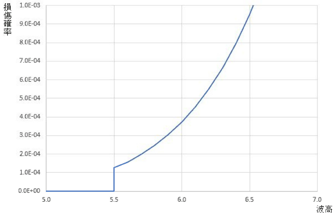
(2) 被水・没水（屋内）のフラジリティ曲線（例：設置 E.L. 5.5m 以下）：拡大図
