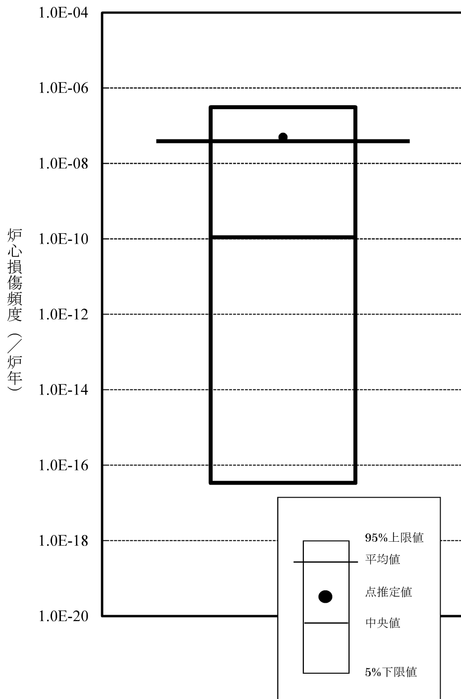
第 3.1.3.2.2.4.8 図 炉心損傷頻度の不確実さ解析結果
