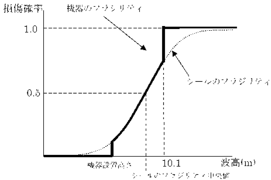
第 3.1.3.2.2.3.2 図 建屋内機器の被水・没水のに関する脆弱性曲線のイメージ
