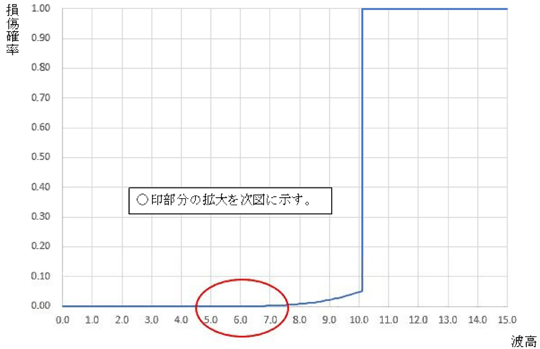
(1) 被水・没水（屋内）のフラジリティ曲線（例：設置 E.L.5.5m 以下）
