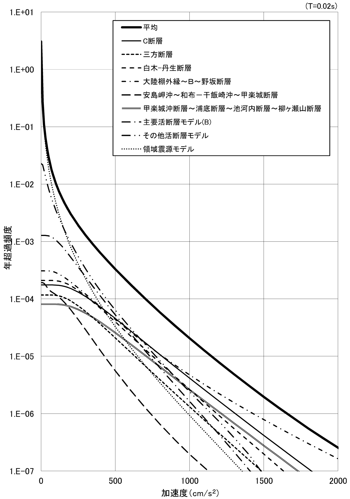
第 3.1.3.2.1.2.7 図 震源ごとのハザード曲線 (周期 0.02 秒)
