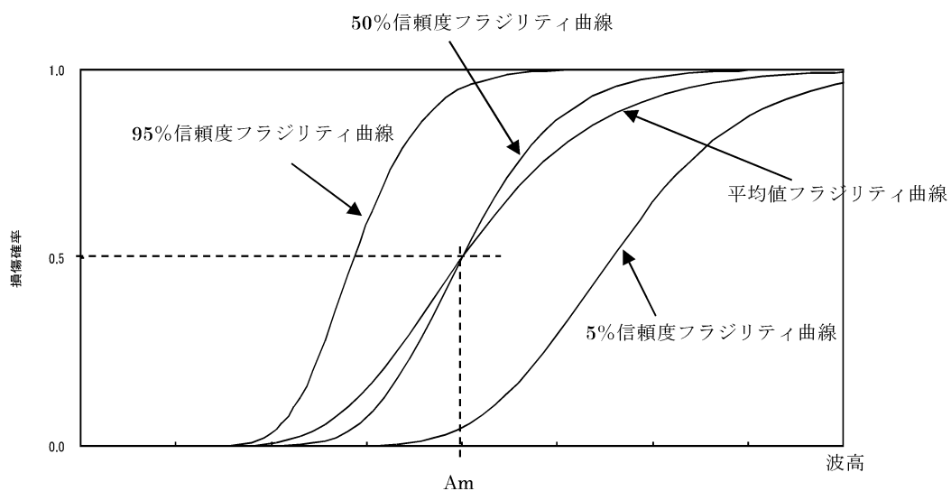
第 3.1.3.2.2.3.3 図 信頼度に応じた脆弱性曲線のイメージ
