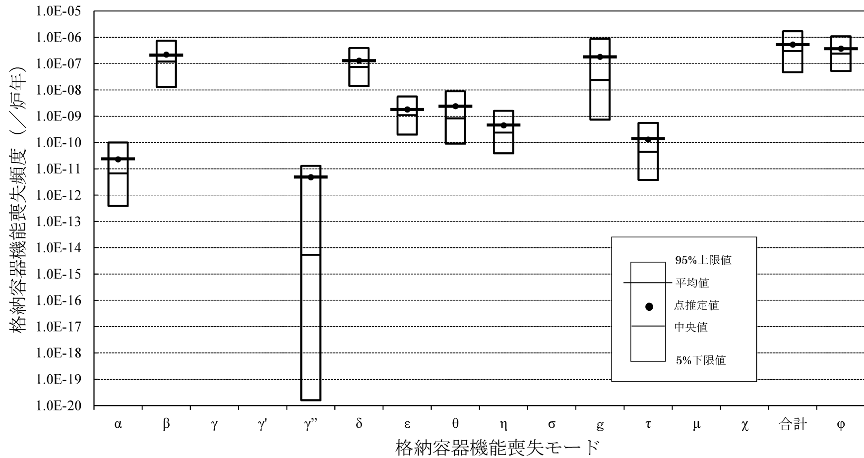
第 3.1.3.2.1.5.4 図 格納容器機能喪失頻度の不確実さ解析結果 (格納容器機能喪失モード別)
