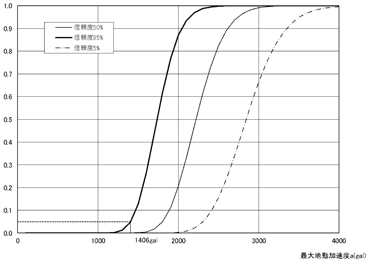
第 3.1.3.2.1.3.14 図 建屋フラジリティ曲線 (原子炉補助建屋)
