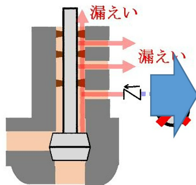
SBO時の1次冷却材の流れ (SDSなし)
