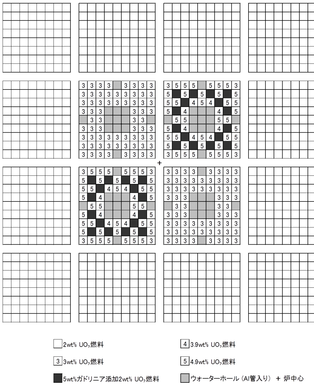
図 4.2-19 NCA 臨界試験体系列 (高温模擬試験)
