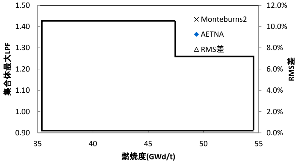
図 4.3-30 制御棒履歴運転時燃料棒最大 LPF 及び RMS 差 (D 格子 9 × 9 燃料)
