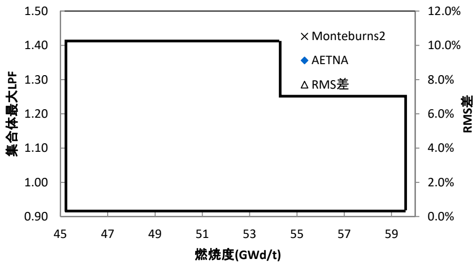
図 4.3-31 制御棒履歴運転時燃料棒最大 LPF 及び RMS 差 (C 格子 10 × 10 燃料)
