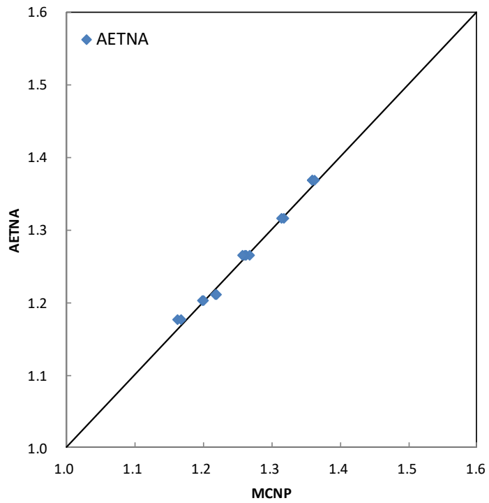
図 4.3-10 初装荷多種類燃料炉心問題の燃料集合体最大 LPF の比較 (炉心 1)
