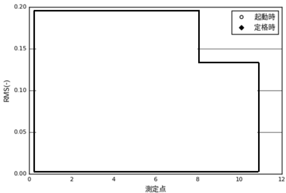
図 4.3-88 TIP 測定値と計算値の径方向 RMS 差 (部分出力運転)
