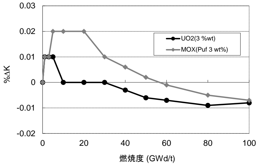
図 3.1-9 FP チェーンモデルの不確かさ
