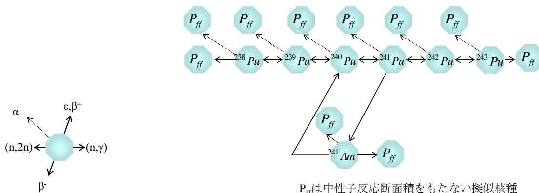
図 3.1-16 プルトニウム起源対象核種チェーン
