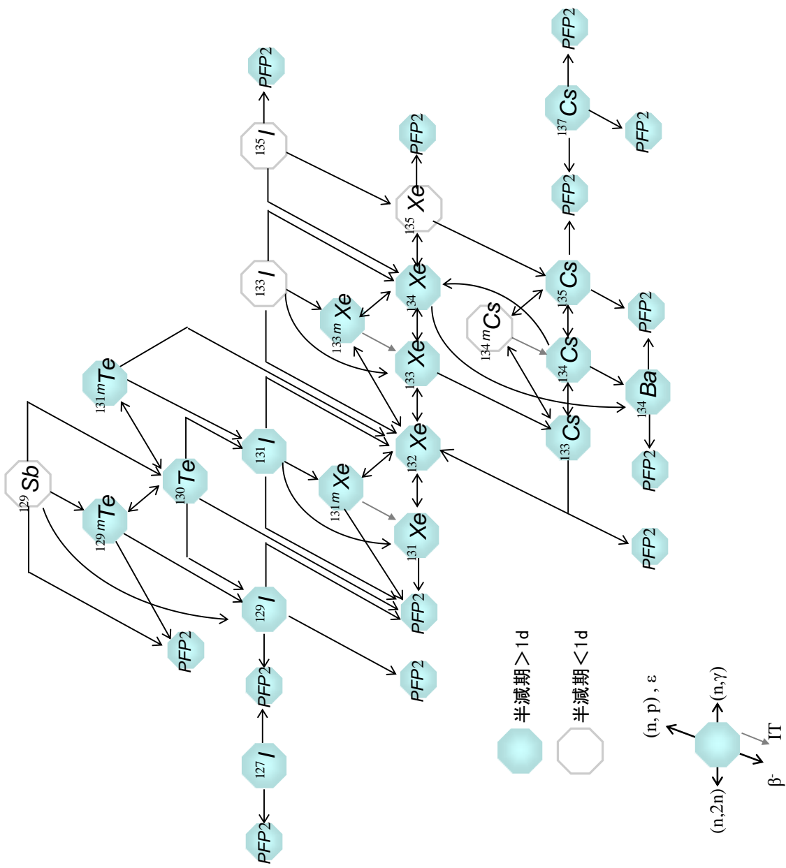
図 3.1-13 核分裂生成核種の生成・崩壊チェーン (その 2)
