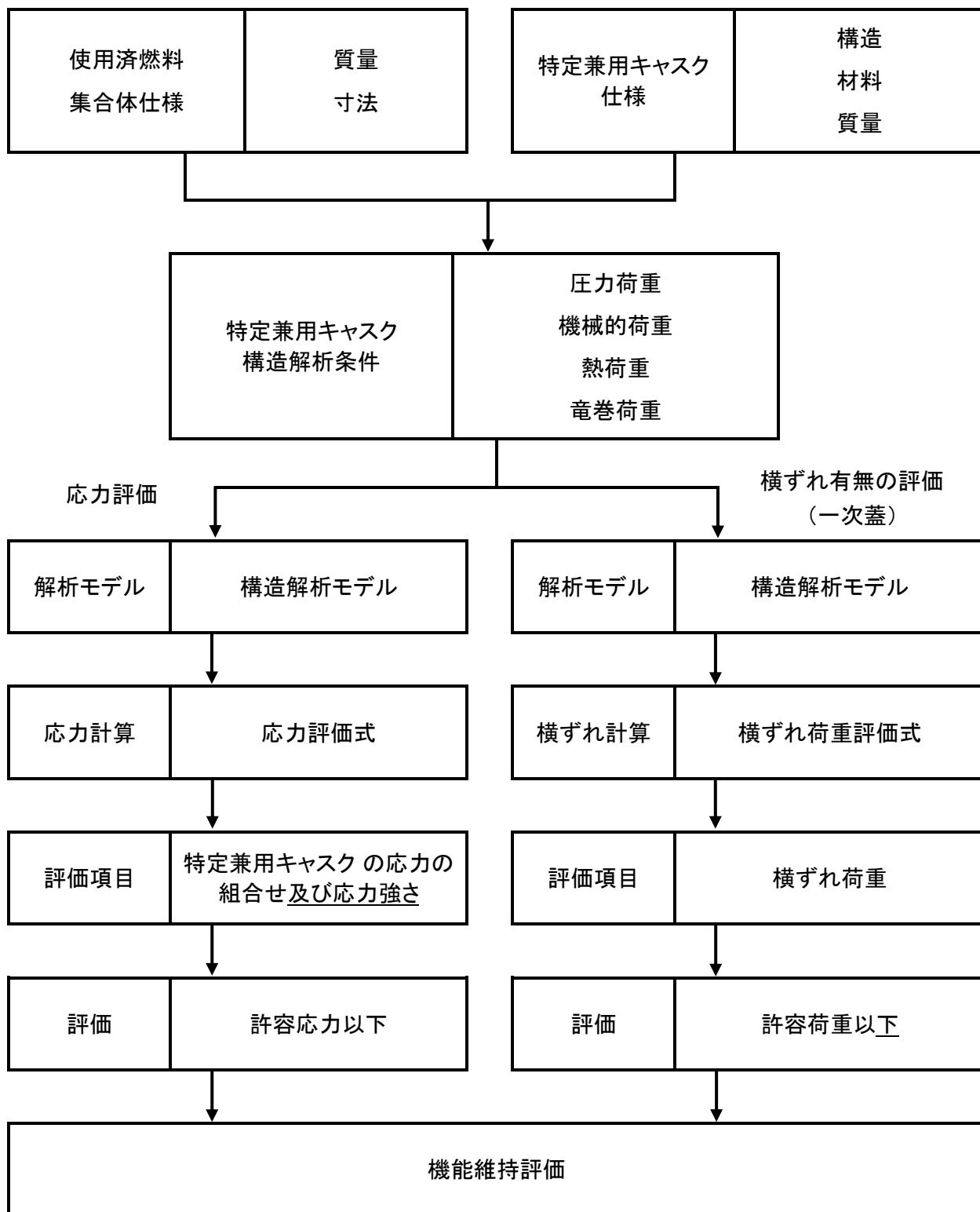
図 1: 竜巻荷重作用時の機能維持評価フロー
