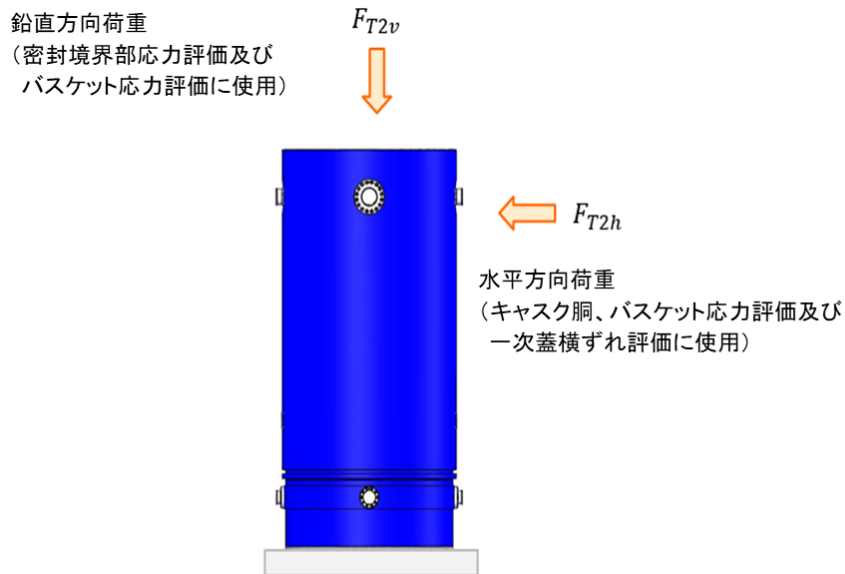
図 A-1 竜巻荷重の作用方向
