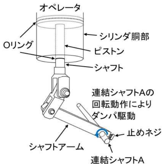
ダンパ駆動部模式図
