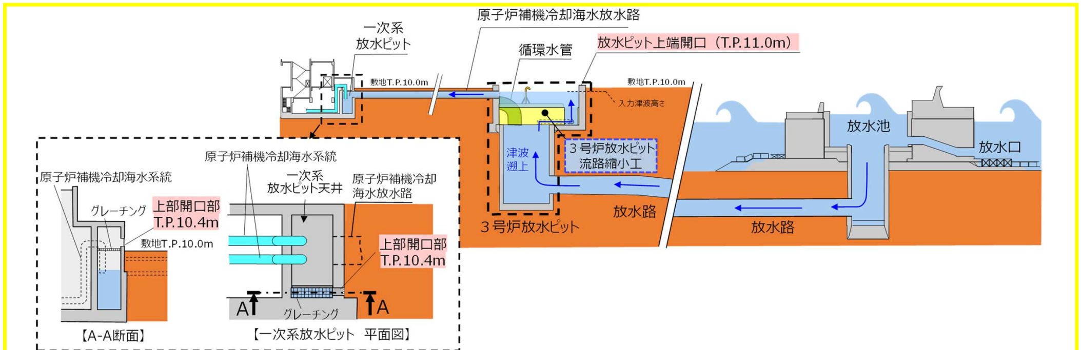
図4 3号炉放水ピット流路縮小工設置イメージ図
