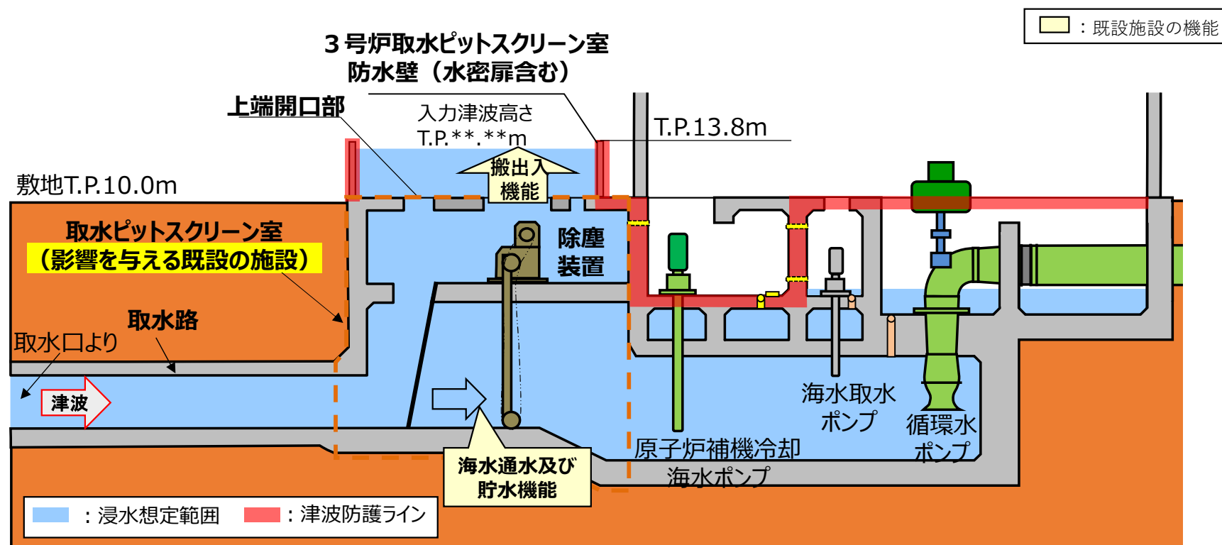
図2 3号炉取水系断面図
