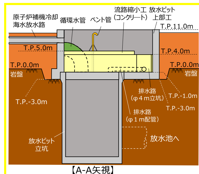
図5 3号炉放水ピット流路縮小工の構造概要図
