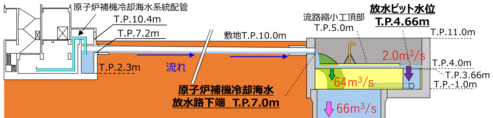
図10 流路縮小工施工後の3号炉原子炉補機冷却海水系統の排水経路
