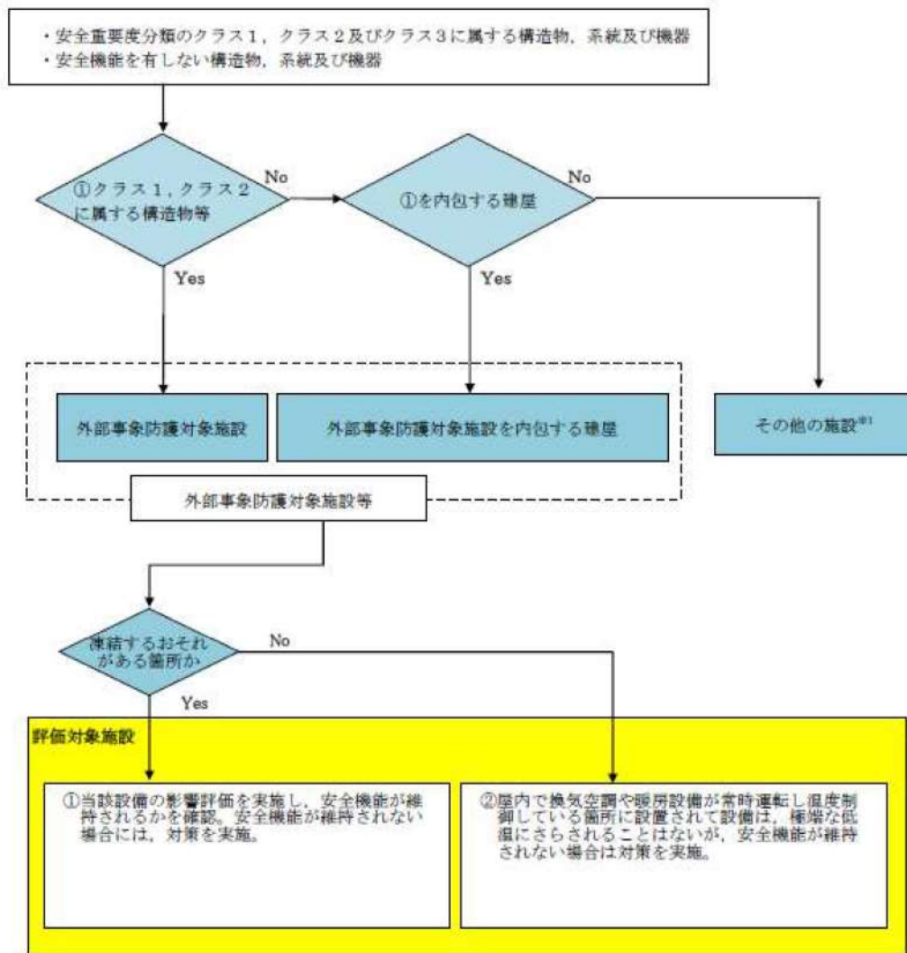
第1図 凍結に対する安全施設の評価フロー
