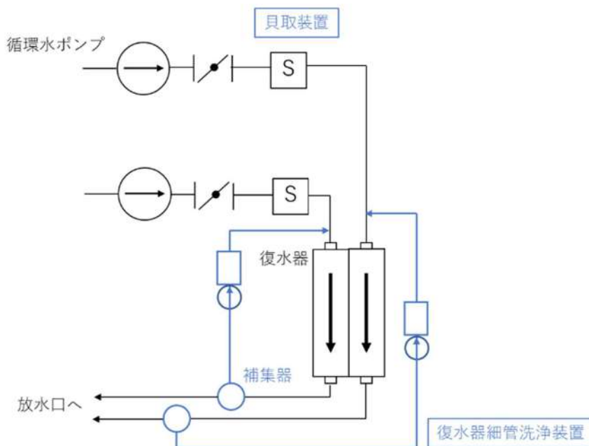
第8図 循環水設備略 6条自然-別1-補7
