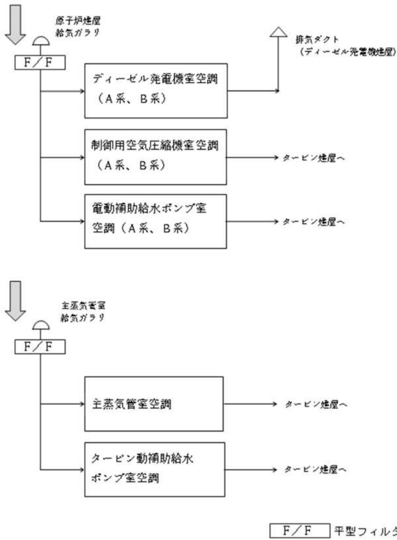
図 8-2(c) 原子炉建屋換気空調設備全体概要図
