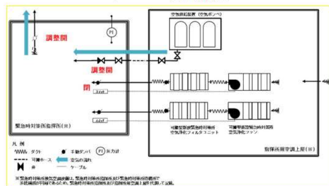
緊急時対策所加圧設備による正圧化時の気密性, 正圧化機能に関する 試験・検査性 概略図(プルーム通過中)
