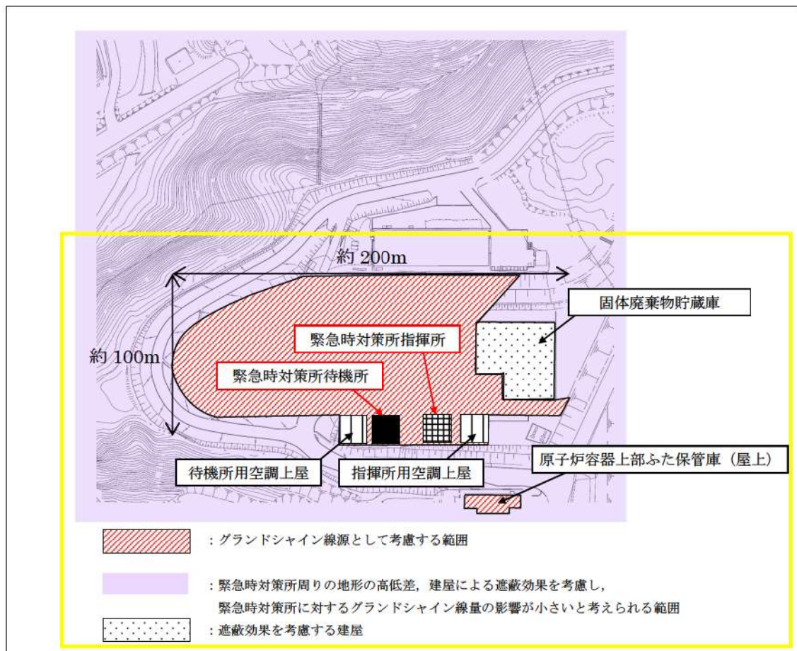
図添9-1 緊急時対策所のグラントシャインガンマ線量評価において考慮する線源範囲
