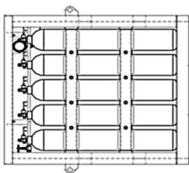
空気供給装置概略図
