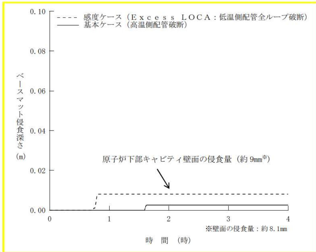
第 7.2.5.8 図 ベースマット侵食深さ (壁面) の推移 (低温側配管全ループ破断時の影響確認)
