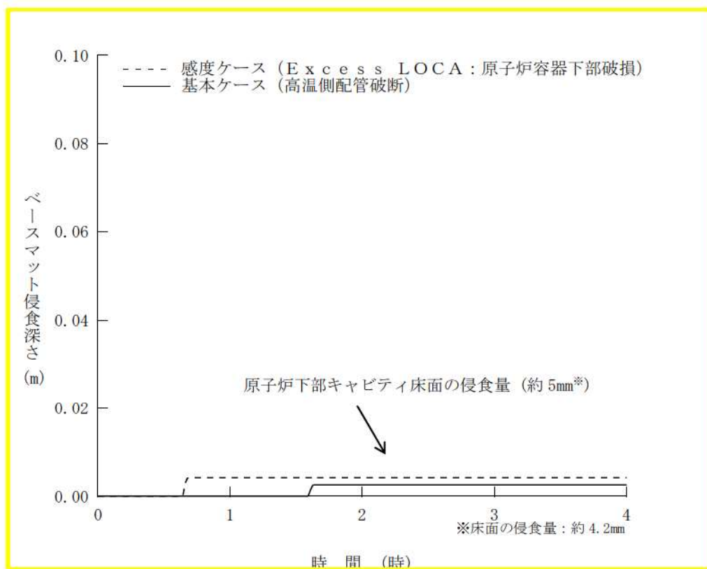
第 7.2.5.10 図 ベースマット侵食深さ (床面) の推移 (原子炉容器下端における破損時の影響確認)
