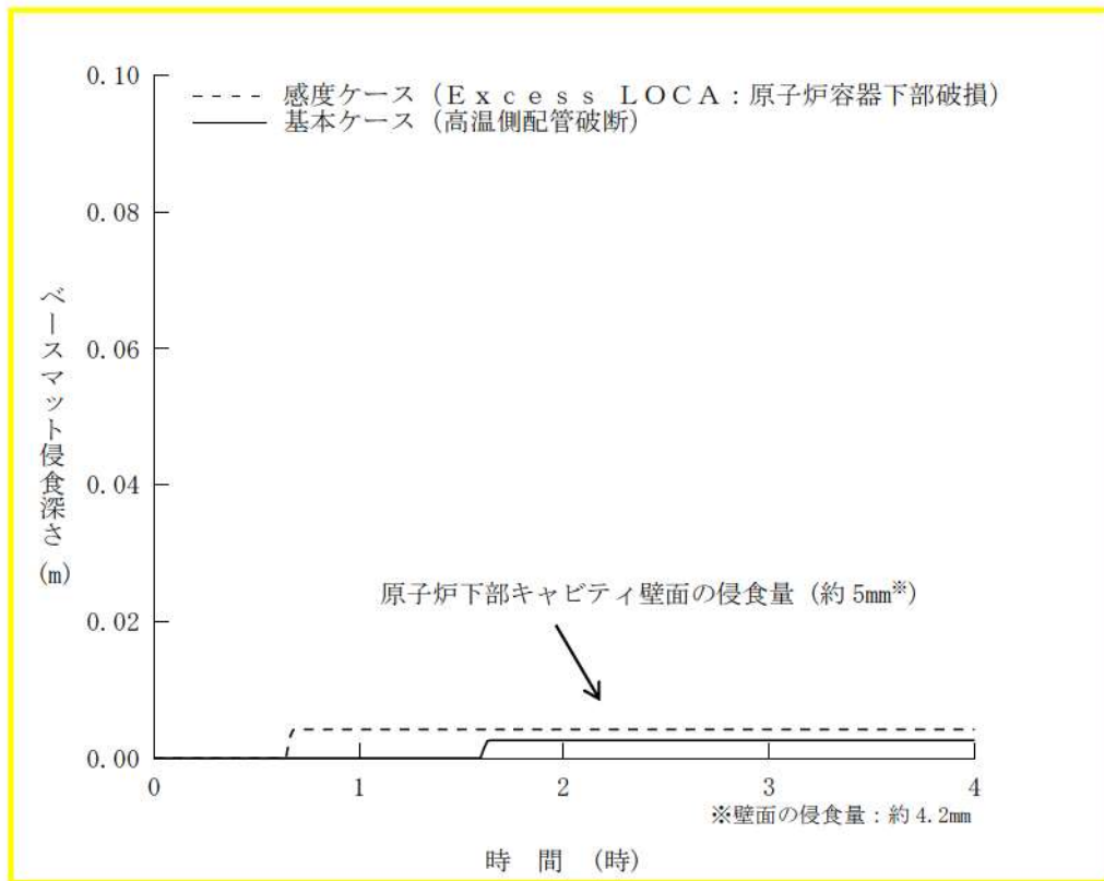
第 7.2.5.11 図 ベースマット侵食深さ (壁面) の推移 (原子炉容器下端における破損時の影響確認)
