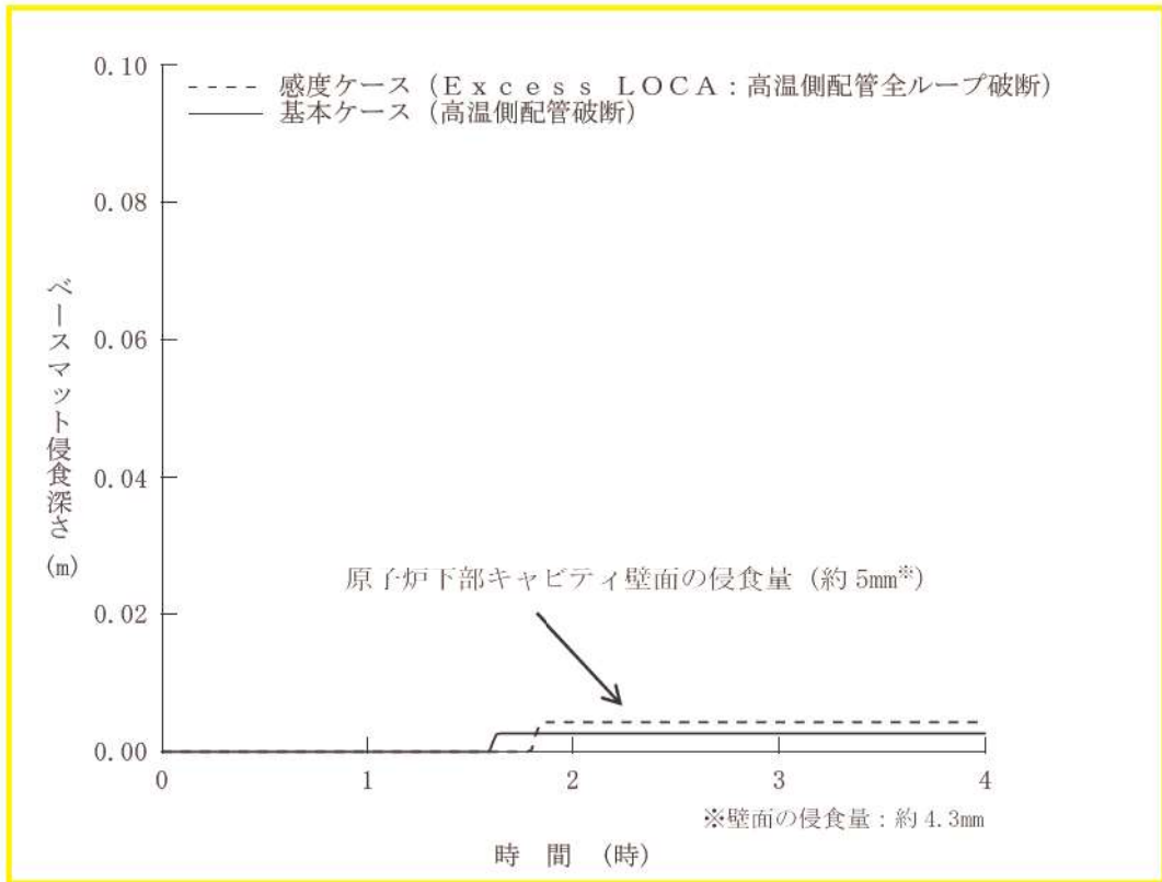
第 7.2.5.5 図 ベースマット侵食深さ (壁面) の推移 (高温側配管全ループ破断時の影響確認)
