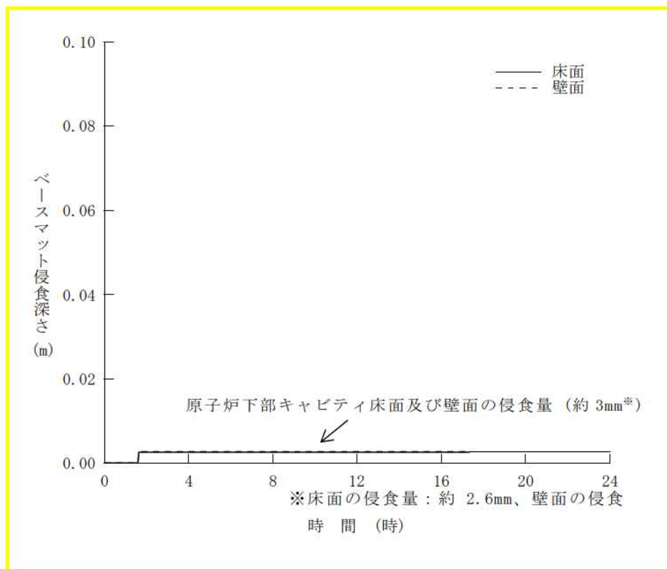
第 7.2.5.2 図 ベースマット侵食深さの推移
