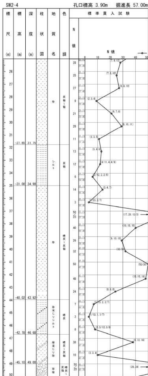
添付 1-2 図(2/3) ボーリング柱状図・コア写真 (SW2-4)
