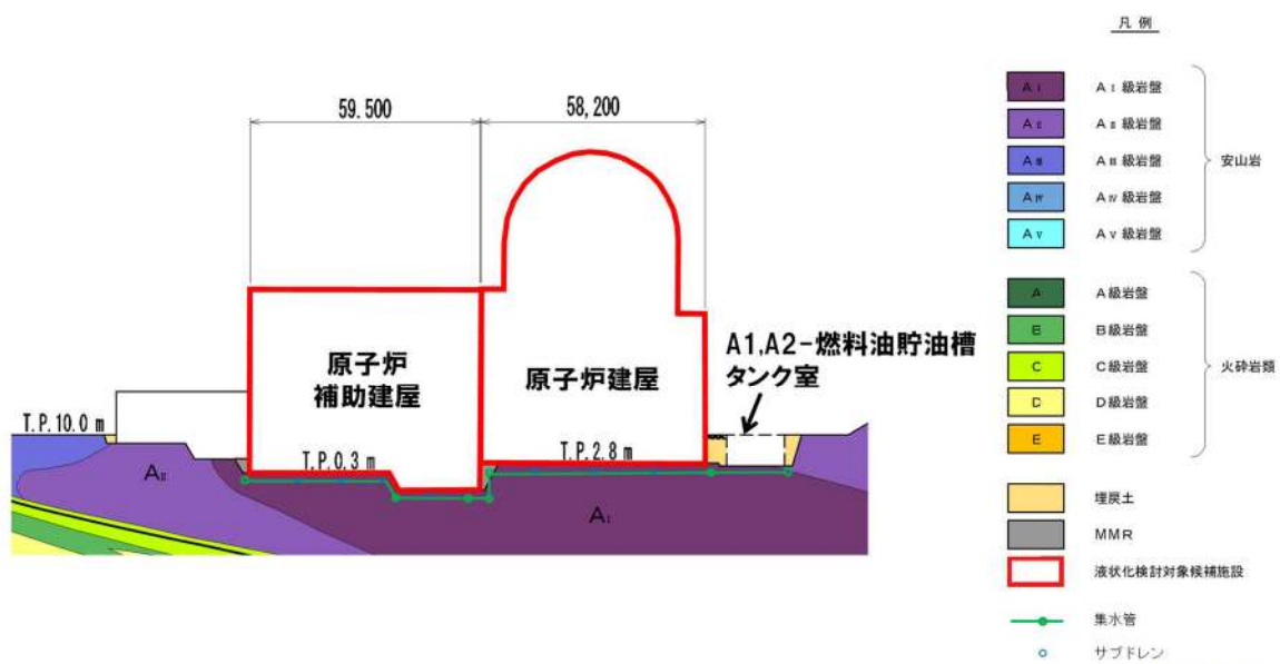
第 3.2-1 図 原子炉建屋，原子炉補助建屋，A1, A2-燃料油貯油槽タンク室断面図 (①-①')
