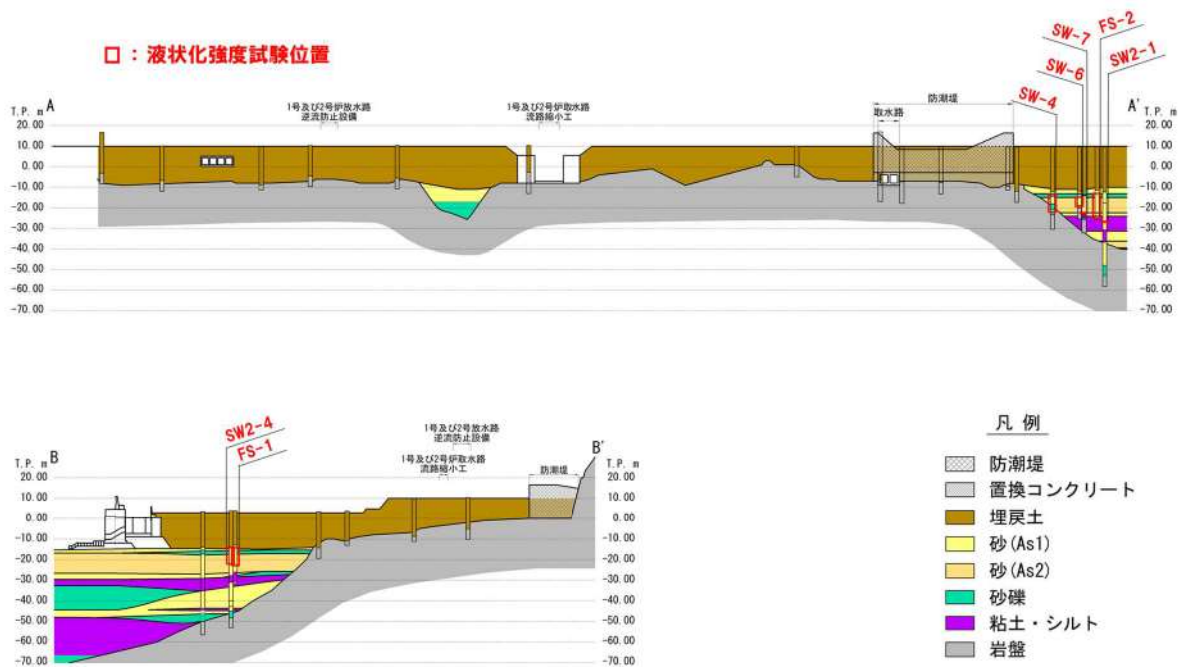
第 4.1-5 図 液状化強度試験に用いる試料採取位置断面図(砂層)
