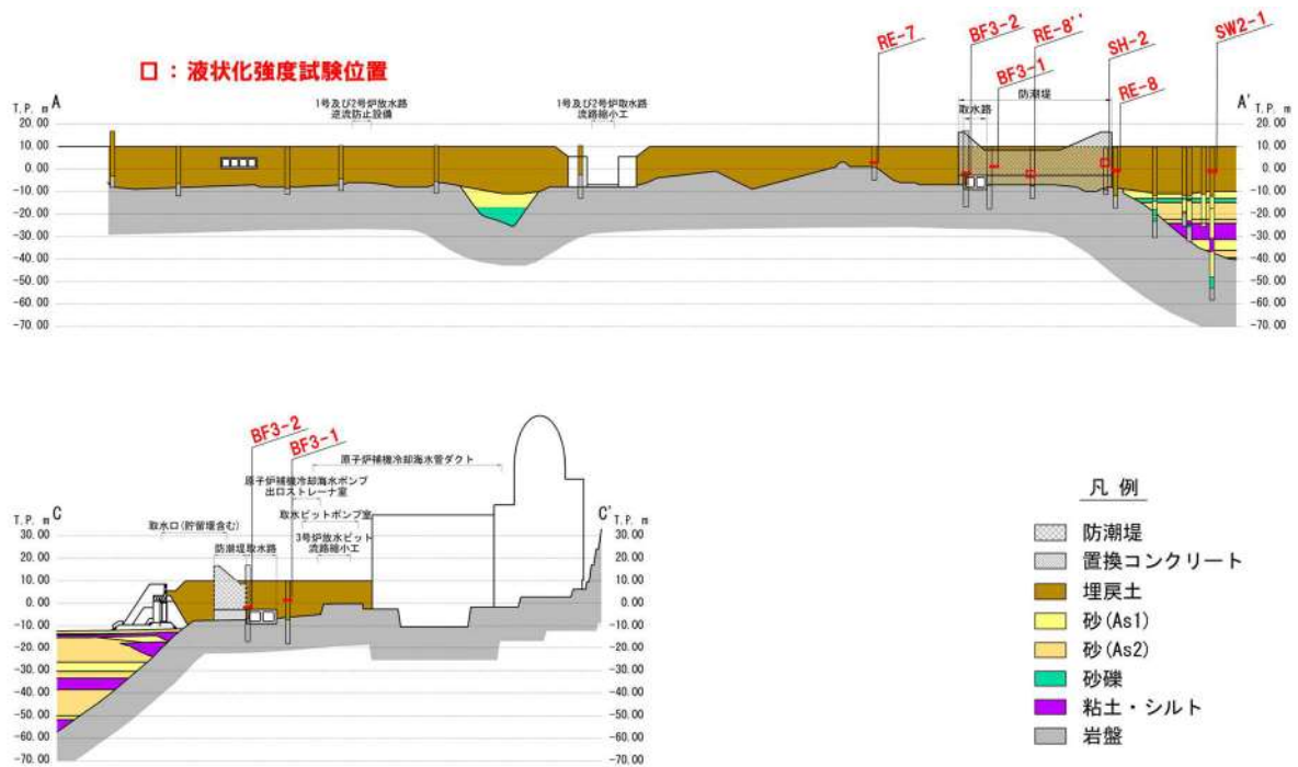
第 4.1-3 図 液状化強度試験に用いる試料採取位置断面図 (3 号埋戻土)
