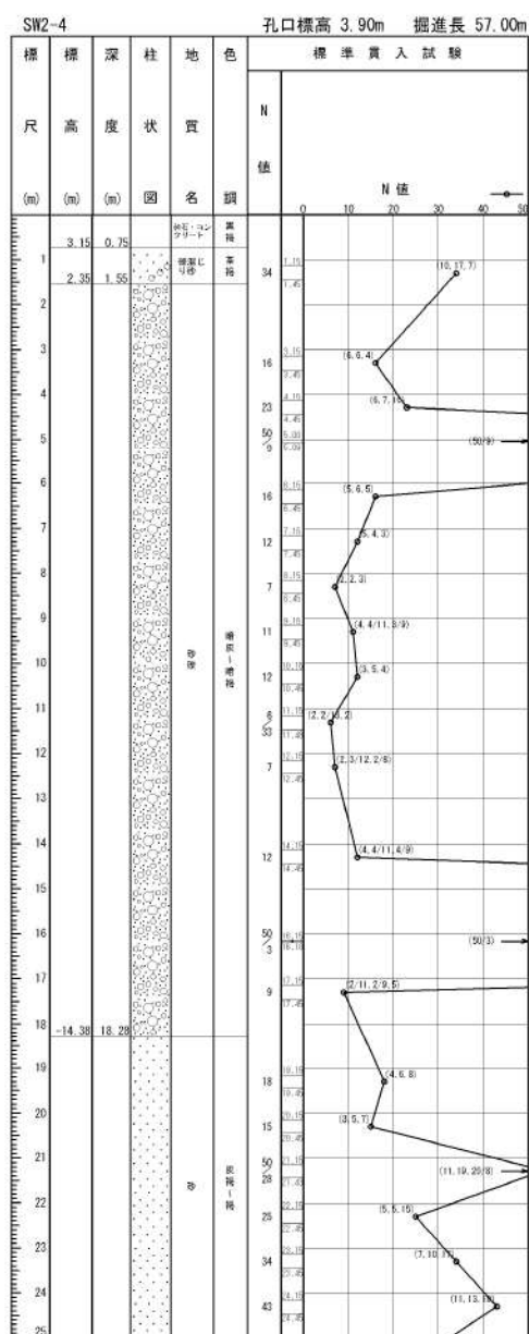
添付 1-38 図(1/3) ボーリング柱状図・コア写真 (SW2-4)
