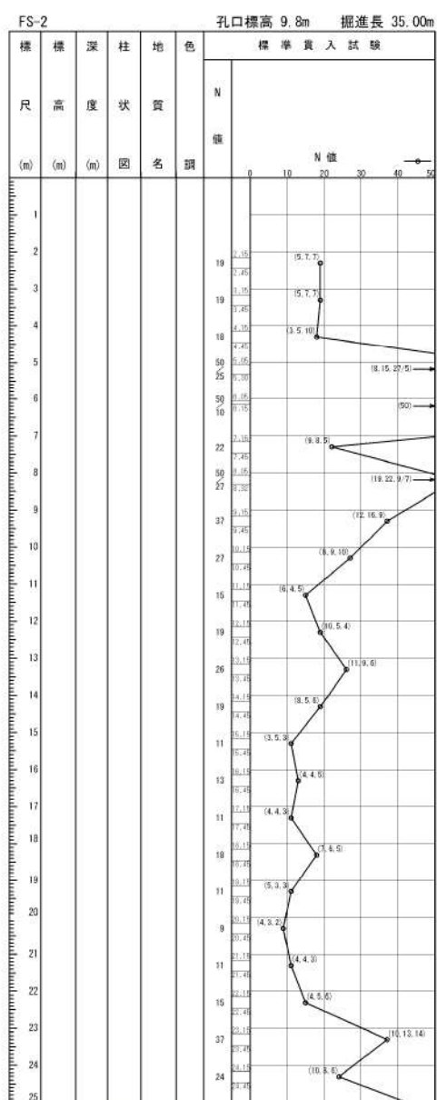
添付 1-40 図(1/10) ボーリング柱状図・コア写真 (FS-2)
