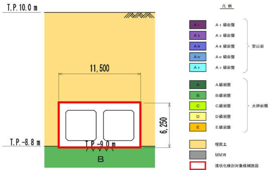
第 3.2-16 図 取水路断面図
