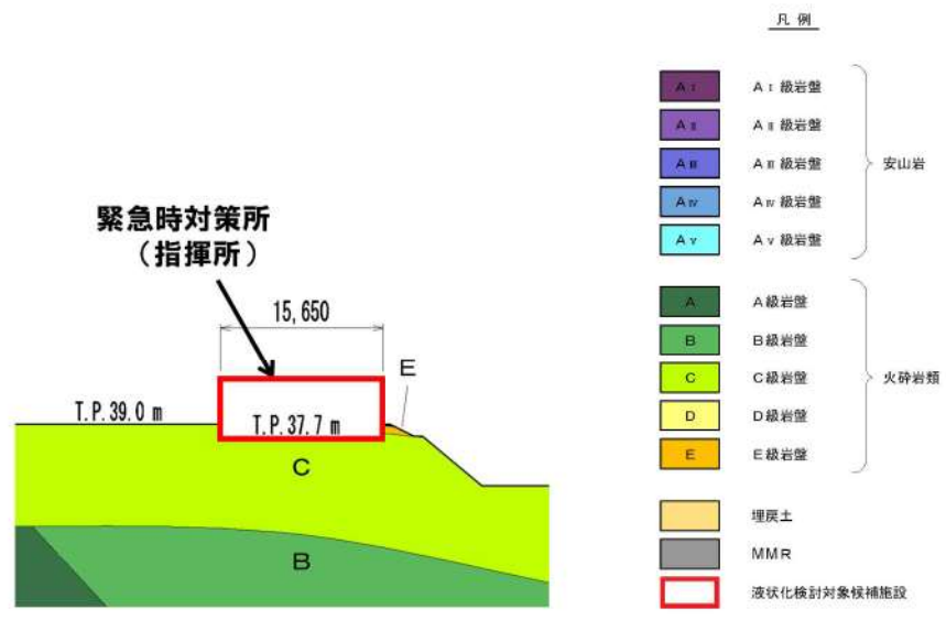
④緊急時対策所(指揮所)断面図(④-④')
