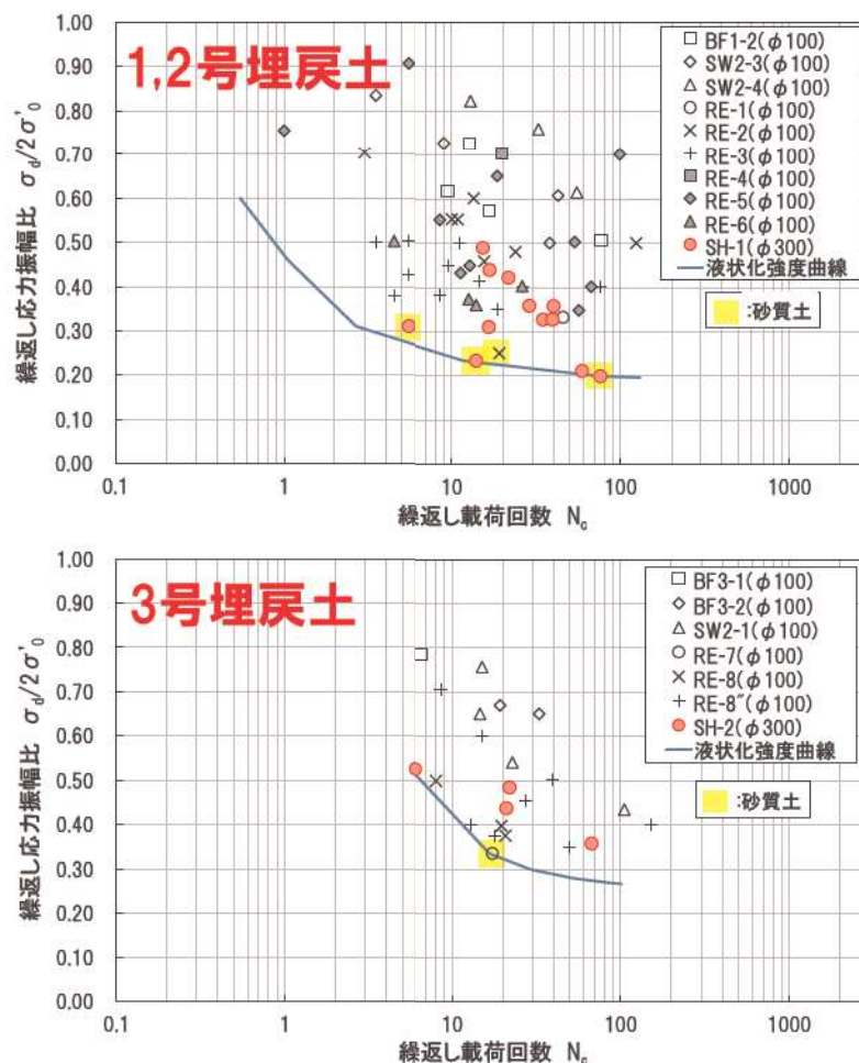
第 5.5-1 図 液状化強度試験結果に基づく埋戻土の液状化強度曲線
