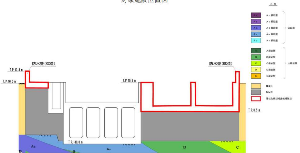
第 3.2-11 図 3 号炉取水ピットスクリーン室防水壁断面図
