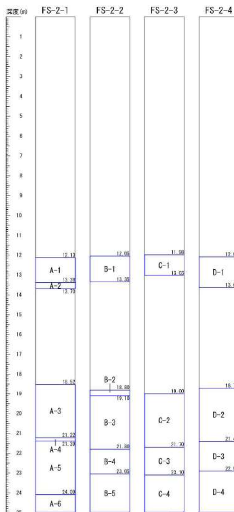
添付 1-40 図(1/10) ボーリング柱状図・コア写真 (FS-2)
