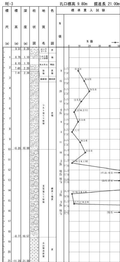
添付 1-6 図 ボーリング柱状図・コア写真 (RE-3)
