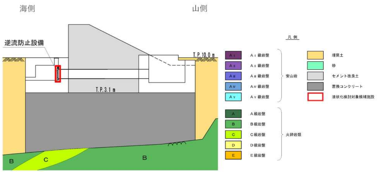
第 3.2-13 図 屋外排水路逆流防止設備断面図
