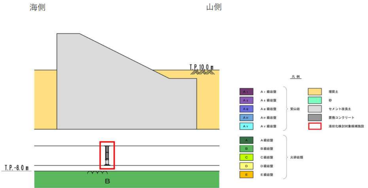
第 3.2-17 図 1 号及び 2 号炉取水路流路縮小工断面図
