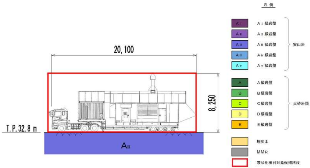
第 3.2-19 図 代替非常用発電機設置位置断面図
