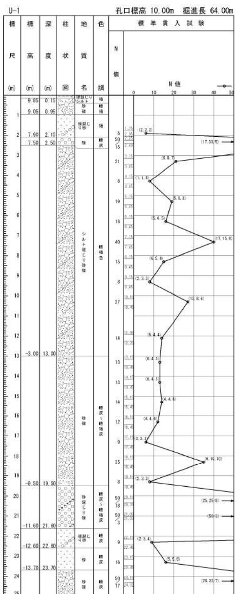
添付 1-41 図(1/3) ボーリング柱状図・コア写真 (U-1)
