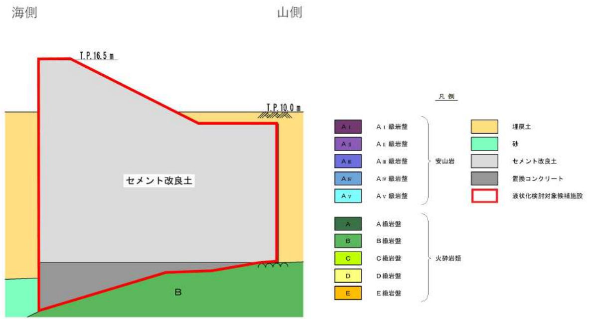
第 3.2-12 図 防潮堤断面図
