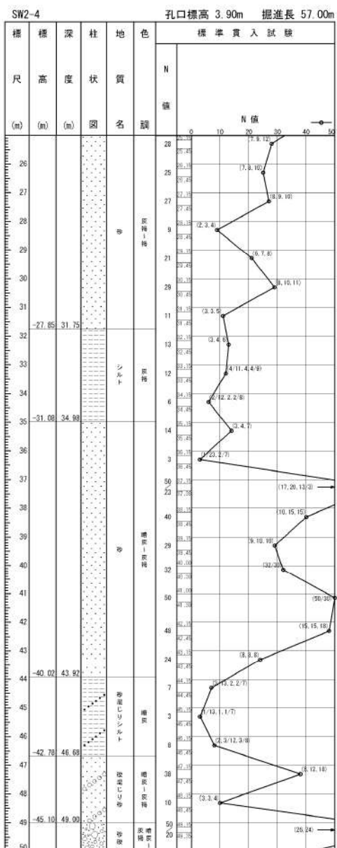
添付 1-38 図(2/3) ボーリング柱状図・コア写真 (SW2-4)
