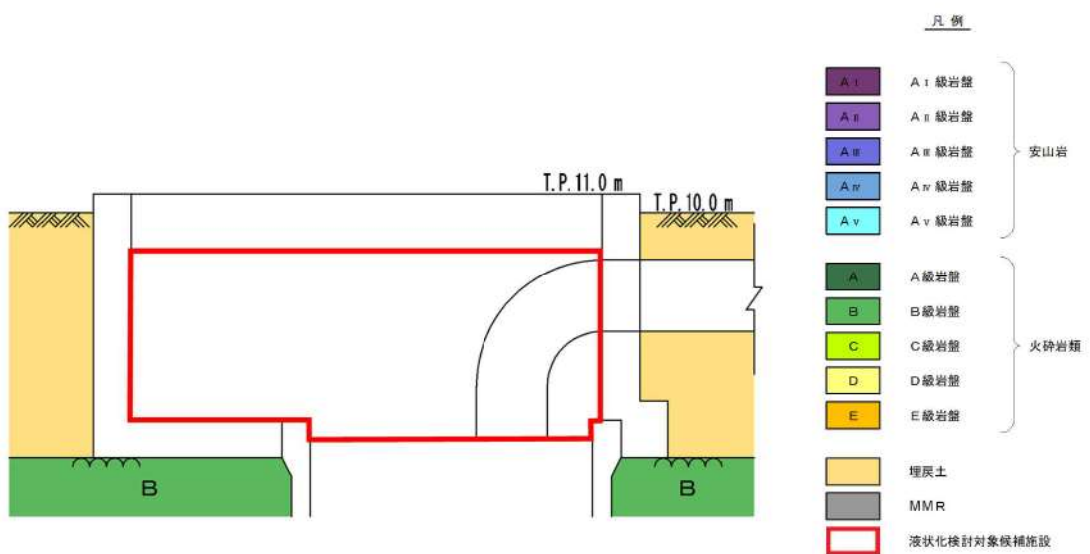
第 3.2-14 図 3号炉放水ピット流路縮小工断面図
