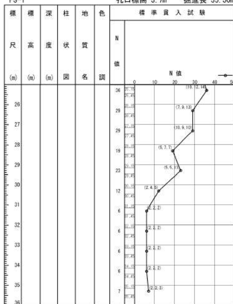
添付 1-39 図(2/10) ボーリング柱状図・コア写真 (FS-1)
