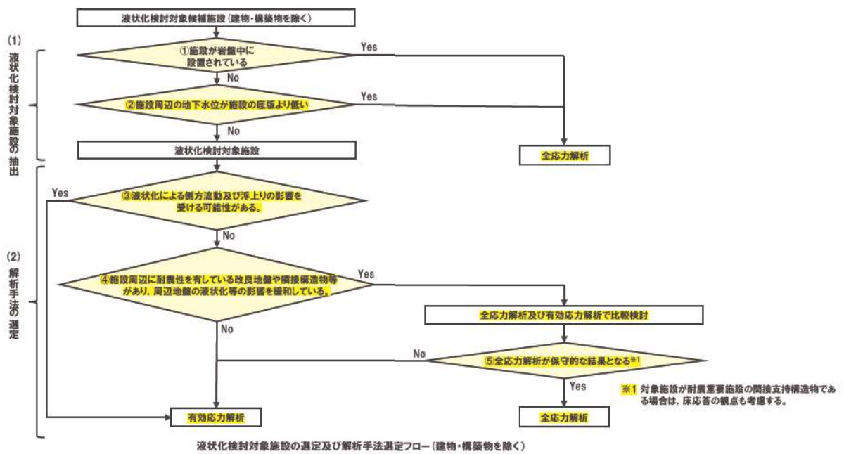
第 3.1-2 図(2) 液状化検討対象施設の選定及び解析手法選定フロー(建物・構築物を除く)
