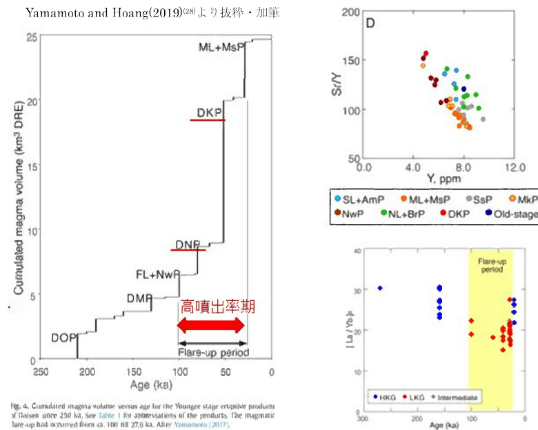
第 1.2.8.3.3 図(2) Yamamoto and Hoang(2019) (28) による大山の噴出率期の評価
