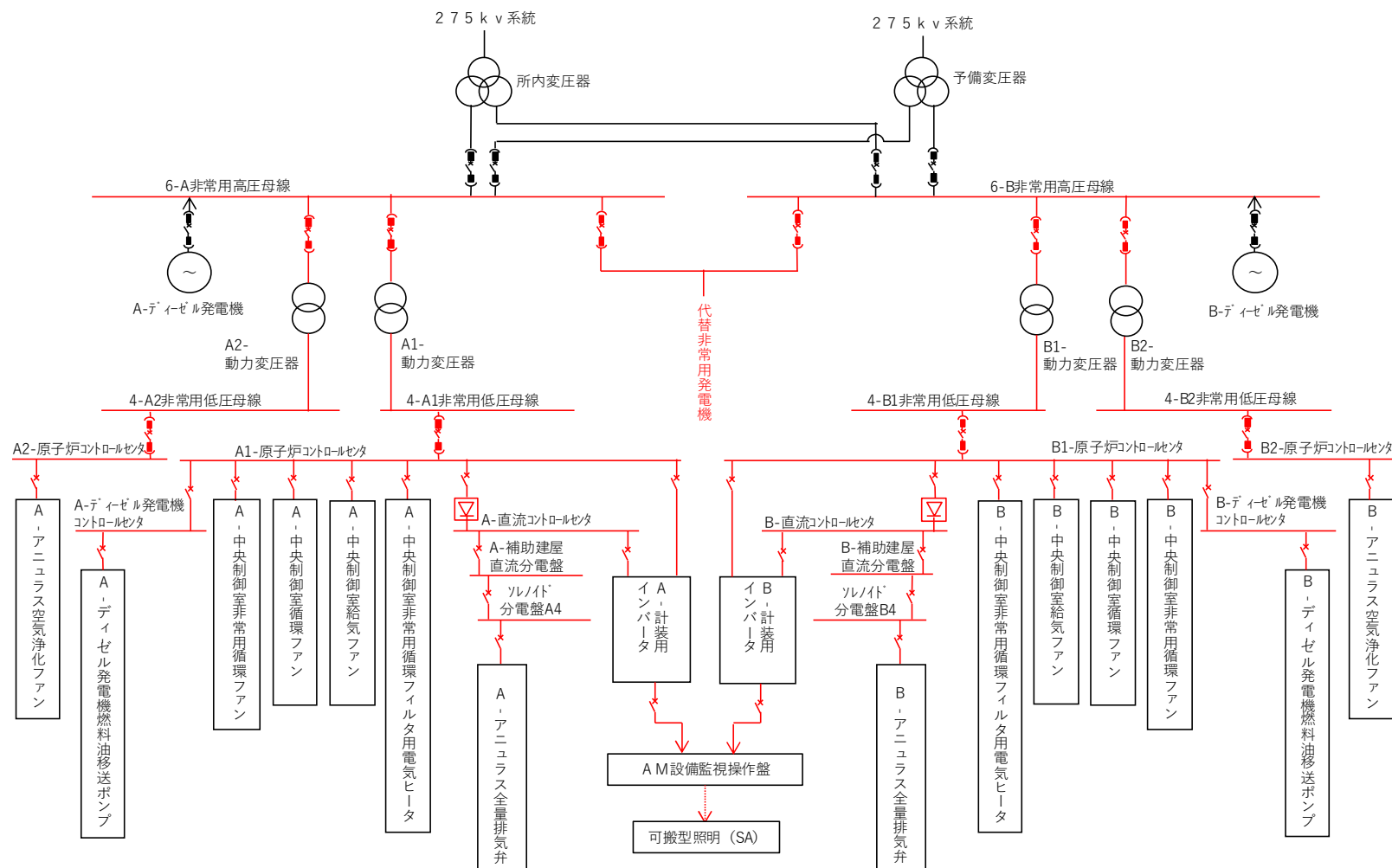
図8 3号炉常設代替交流電源設備系統図 (代替非常用発電機～中央制御室)
