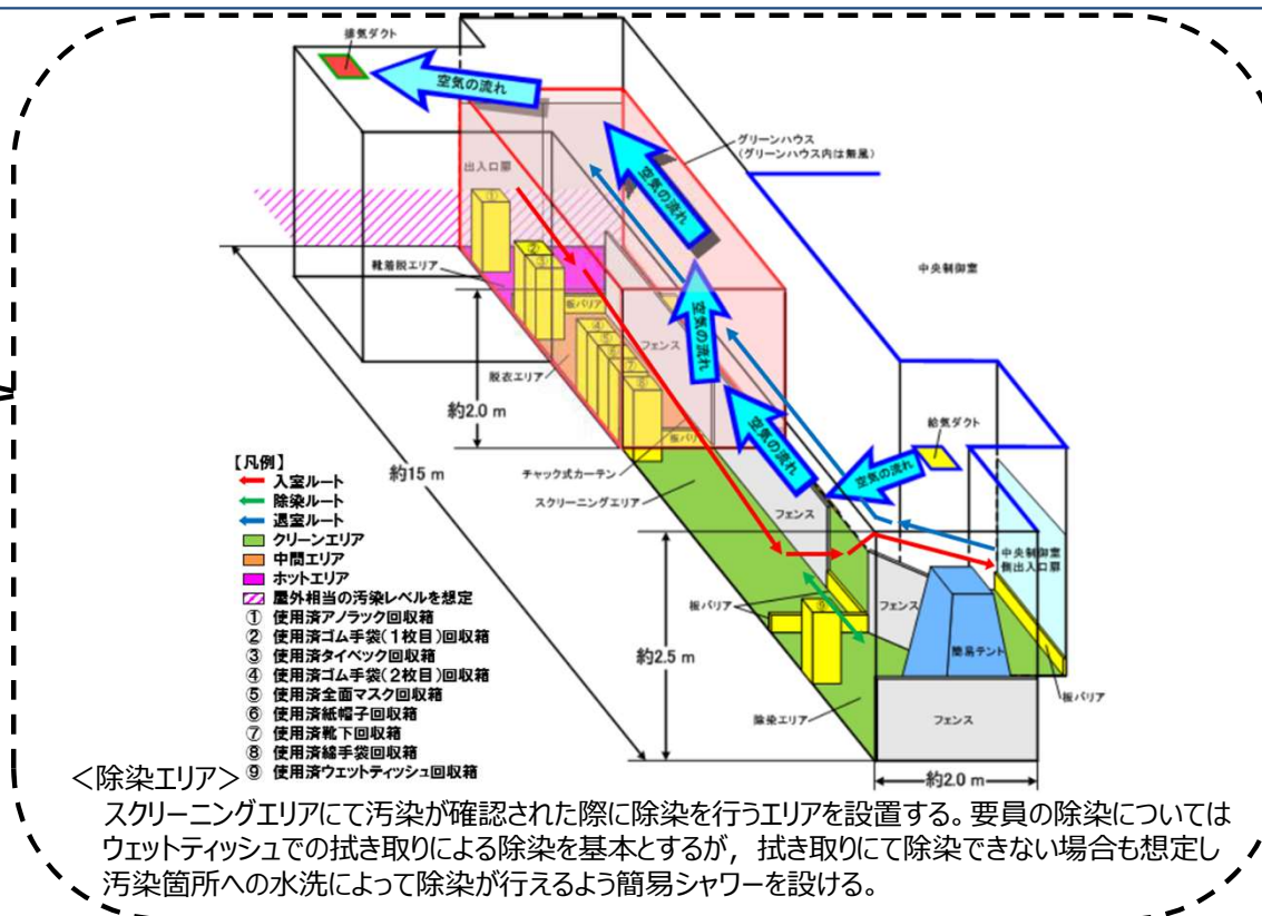
図7 チェンジングエリアのレイアウト
